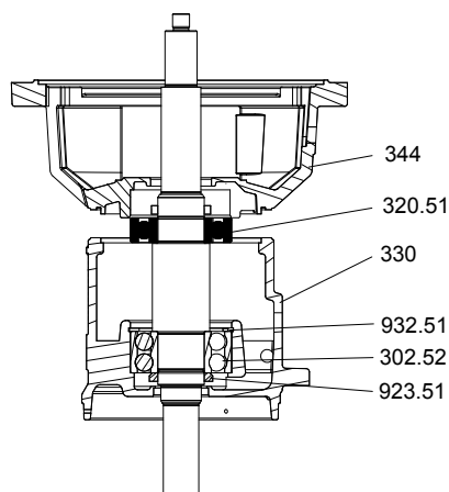
Рис. 37: Поперечное сечение несущей рамы
