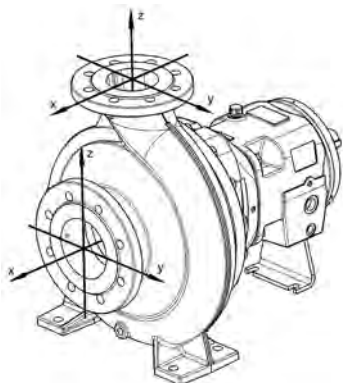
Рис. 20: Внешние силы и моменты на соплах
