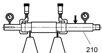
Рис. 42: Проверка прямолинейности
