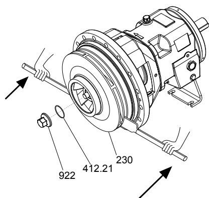
Рис. 33: Способ снятия импеллера
