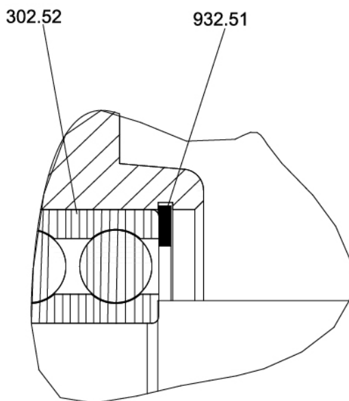
Рис. 49: Деталь стопорного кольца
