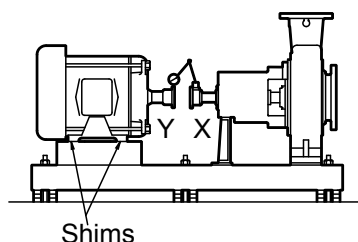
Рис. 16: Неправильная вертикальная соосность (вид сбоку)
