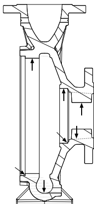
Рис. 38: Участки кожуха, подлежащие осмотру
