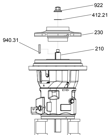
Рис. 34: Компоненты ротора
