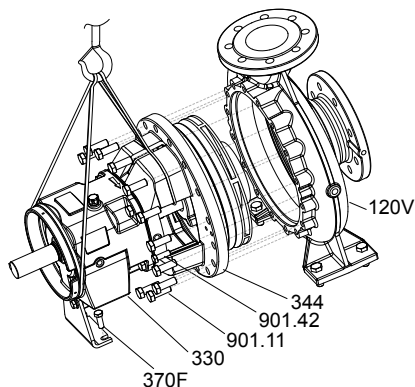
Рис. 51: Установка заднего съемного блока
