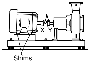
Рис. 14: Неправильная вертикальная соосность (вид сбоку)
