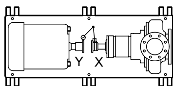
Рис. 17: Неправильная горизонтальная соосность (вид сверху)
