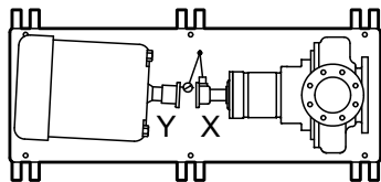
Рис. 15: Неправильная горизонтальная соосность (вид сверху)
