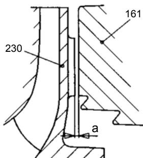
Рис. 32: Проверьте задний зазор
