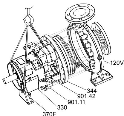
Рис. 30: Проводка каната
