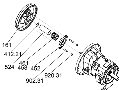
Рис. 36: Снятие уплотнительного и фонарного колец
