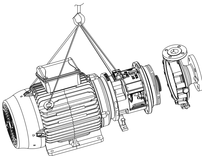
Рис. 31: Задний съёмный узел
