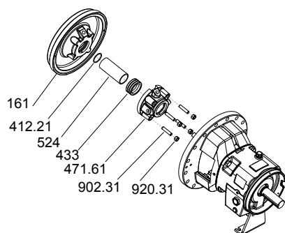
Рис. 35: Снятие сальника
