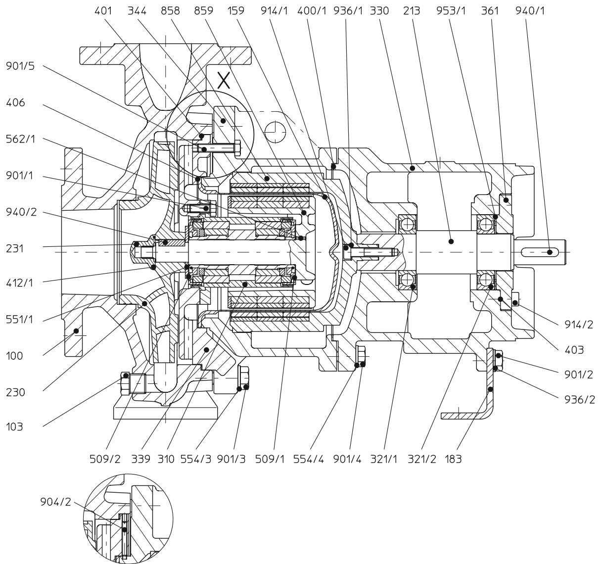
vue en coupe - uniquement avec le groupe 1-160 et 2-160/200
