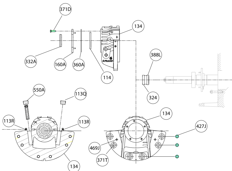
Figura 75: Ensamble del alojamiento de cojinetes radiales
