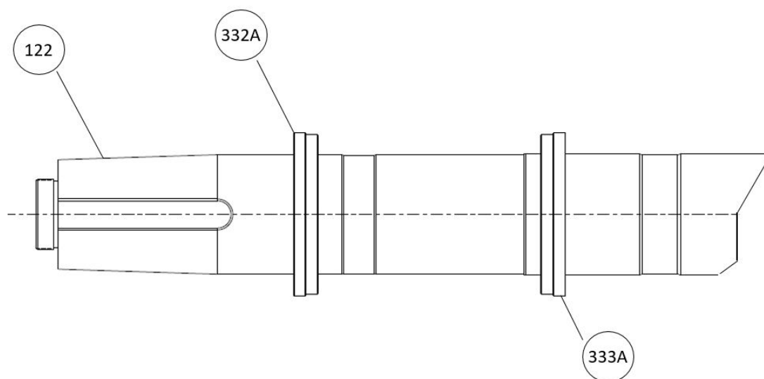
Figura 83: Instalación del sello laberinto radial interno
