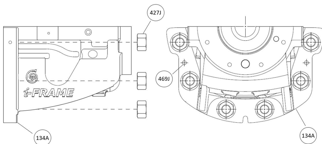
Figura 82: Ensamble el extremo de empuje
