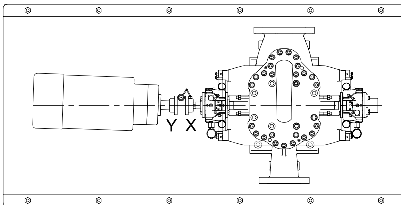
Figura 13: Ejemplo incorrecto de alineación horizontal (vista superior)
