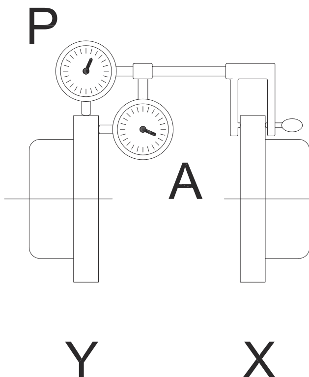
Figura 11: Acoplamiento del indicador de cuadrante
