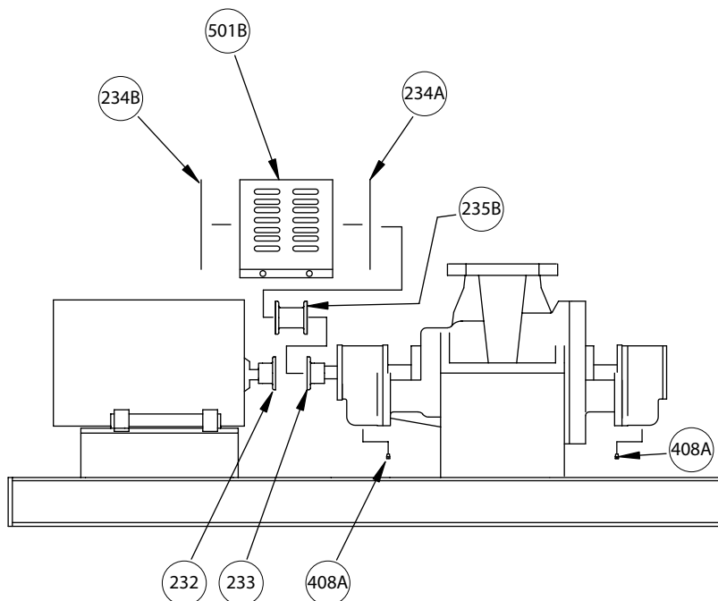
Figura 40: Conjunto del protector del acoplamiento
