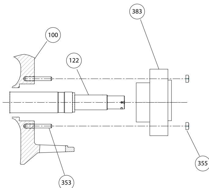
Figura 71: Monte el sello mecánico del cartucho en el extremo de empuje
