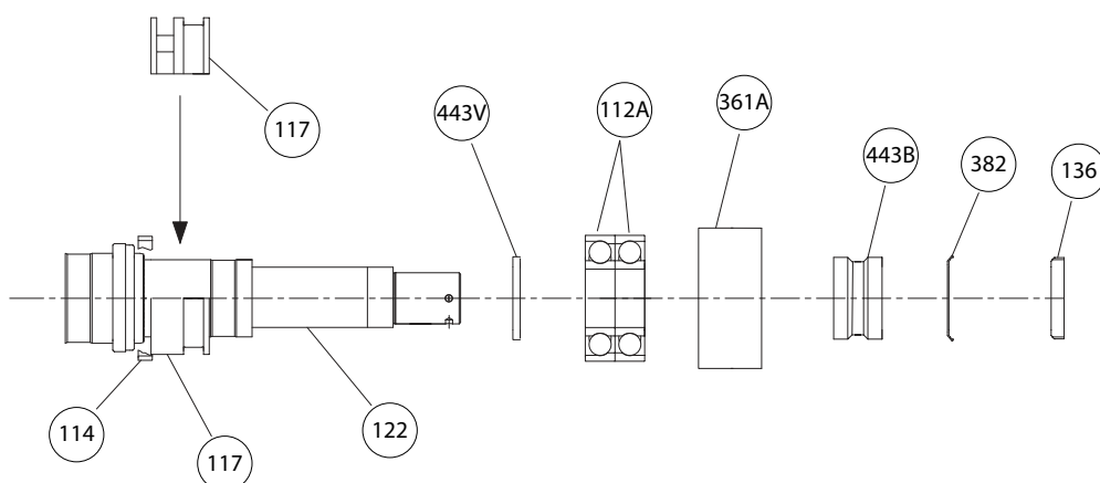
Figura 77: Montaje del manguito y cojinete de empuje
