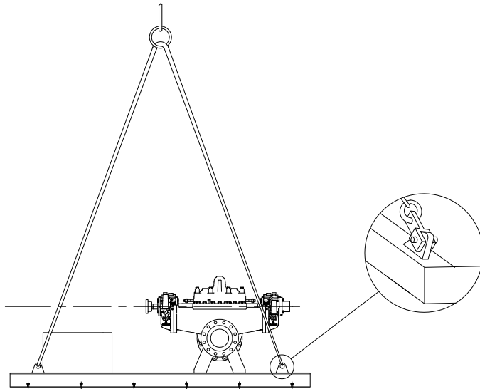
Figura 2: Ejemplo de método de elevación correcto para unidades montadas sobre la plancha de base sin motor con indicación del uso de horquillas
