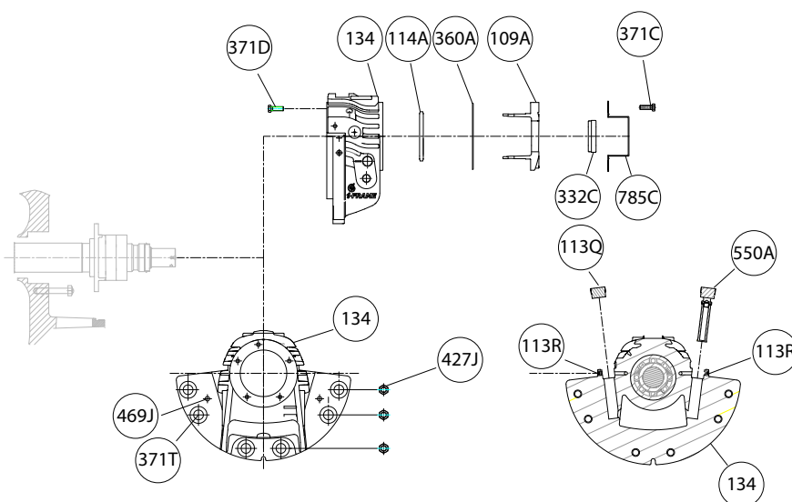
Figura 73: Montaje del bastidor de rodamientos de empuje
