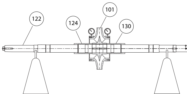
Figura 66: Rotor completamente ensamblado
