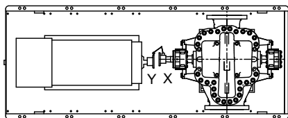
Figura 15: Ejemplo incorrecto de alineación horizontal (vista superior)
