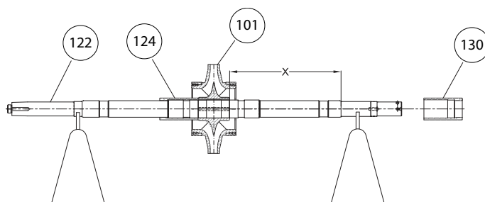
Figura 68: Conjunto del rotor
