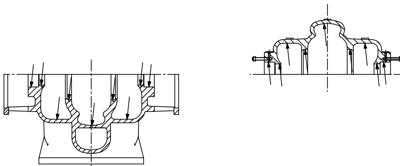
Figura 62: Inspección de la carcasa
