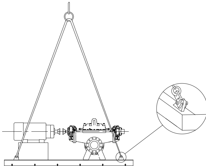
Figura 3: Ejemplo de método de elevación correcto para unidades montadas sobre la plancha de base con motor con indicación del uso de horquillas
