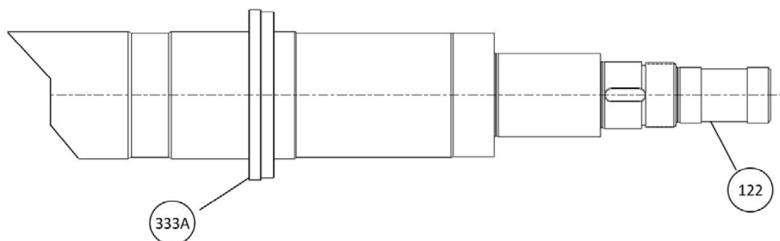
Figura 81: Instalación del sello laberinto de empuje interno
