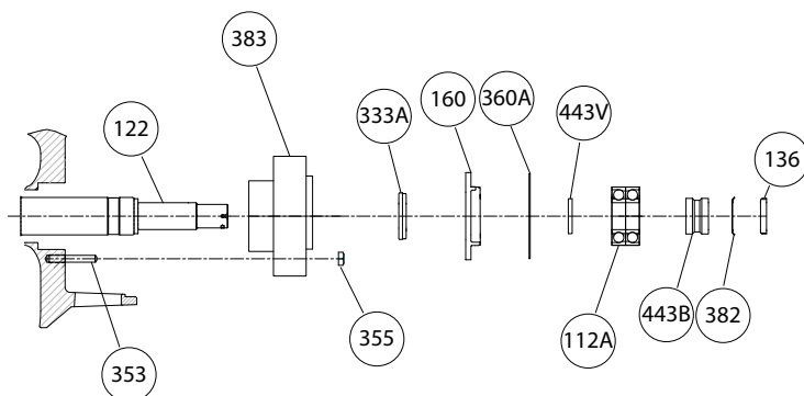
Figura 72: Montaje del cojinete de empuje
