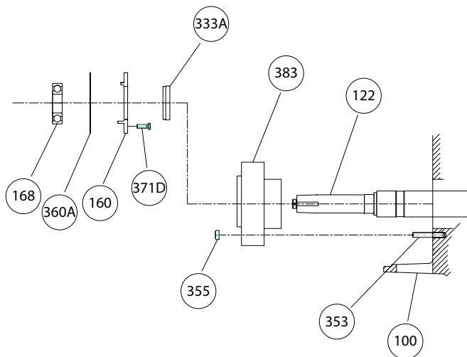
Figura 74: Ensamblaje del rodamiento radial
