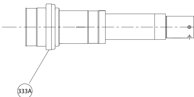
Figura 76: Instalación del sello de laberinto interior
