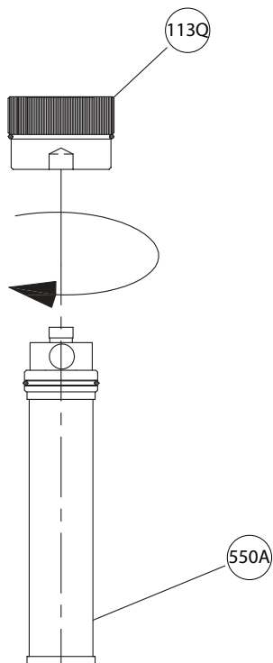
Figura 26: Desmontaje del filtro
