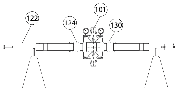
Figura 69: Inspecciones previas al montaje del rotor
