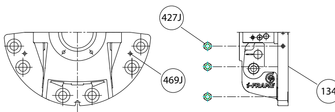
Figura 47: Extracción de la clavija de sujeción
