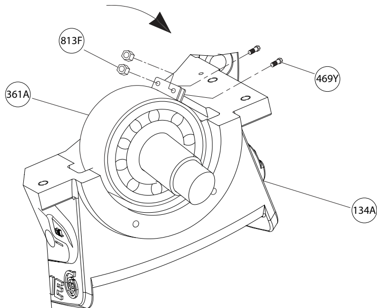
Figura 78: Instalación del retenedor del rodamiento
