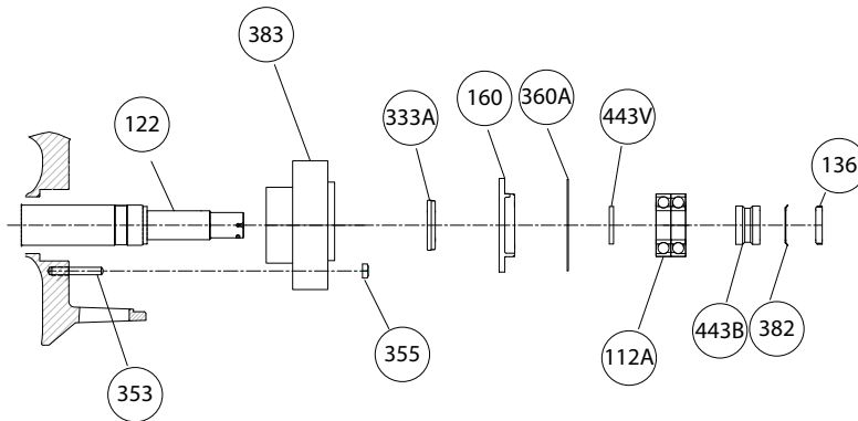
Figura 44: Desmontaje del cojinete de empuje
