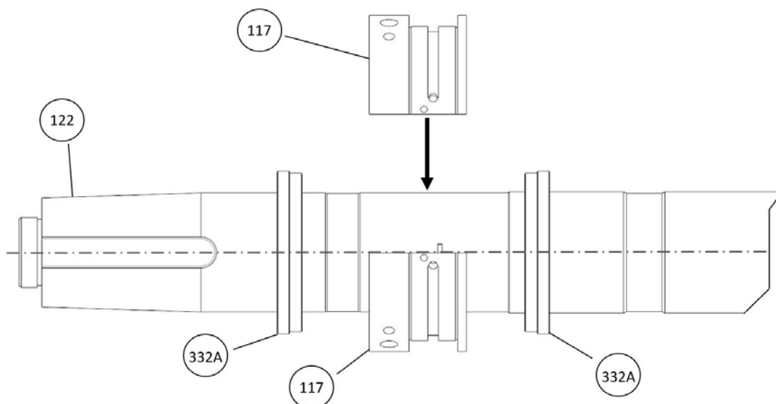
Figura 84: Conjunto de cojinete de manguito radial
