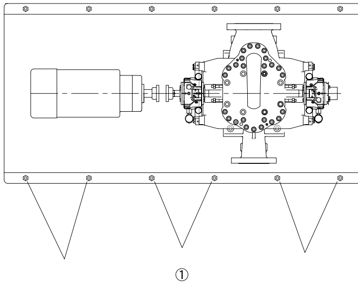
Figura 10: Ubicaciones de los tornillos elevadores, vista superior
