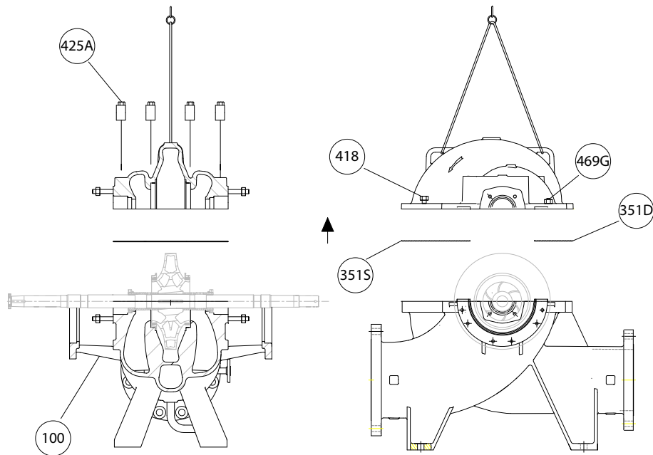
Figura 59: Elimine la mitad superior con una eslinga
