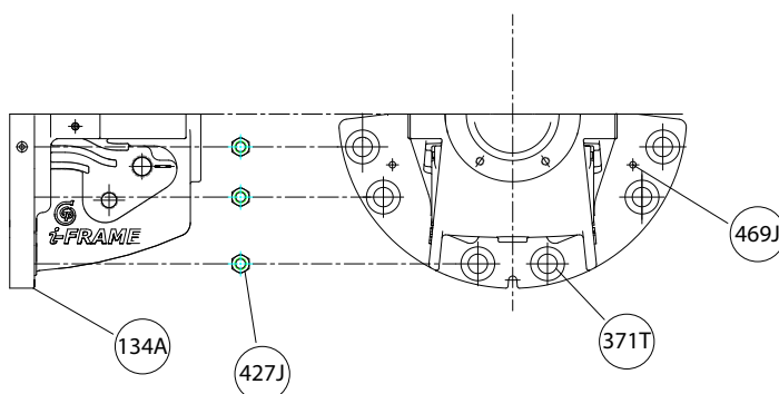
Figura 79: Ensamble la mitad inferior de bastidor de cojinetes
