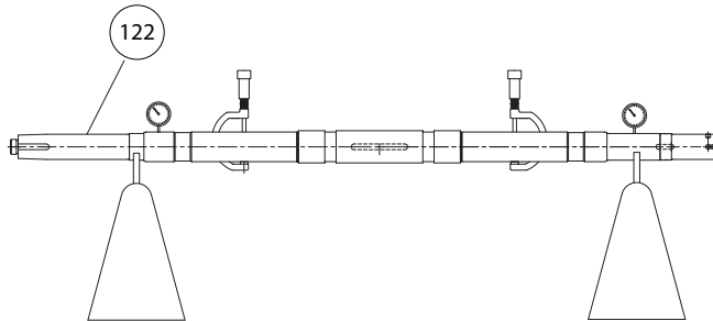
Figura 65: Inspección del eje
