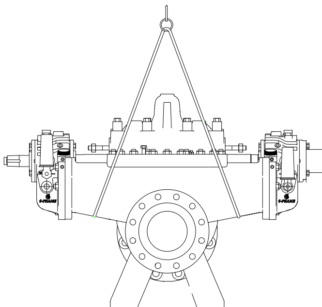
Figura 1: Ejemplo de método de elevación correcto para una bomba vacía
