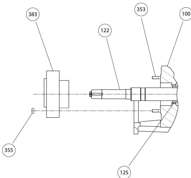
Figura 70: Monte el sello mecánico del cartucho en el extremo radial
