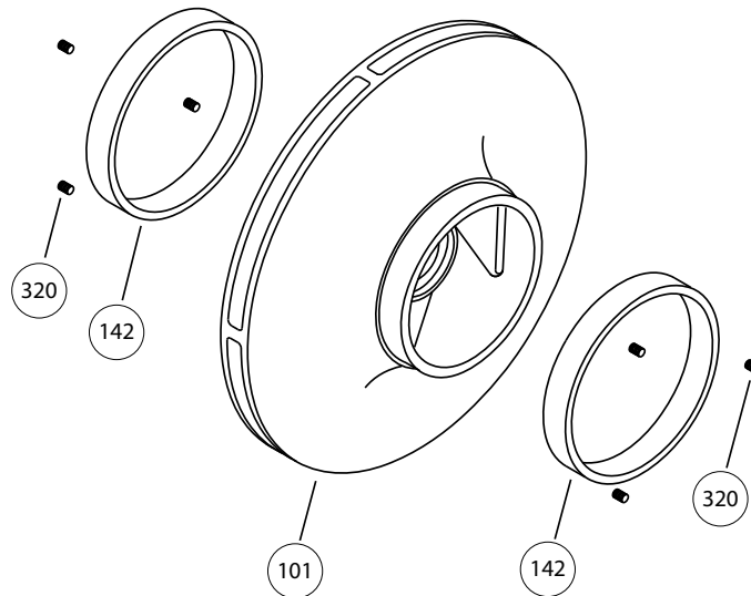
Figura 67: Reemplazamiento del anillo de desgaste
