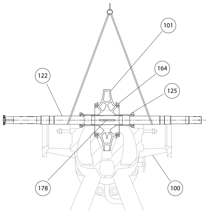
Figura 60: Retiración del rotor de la bomba
