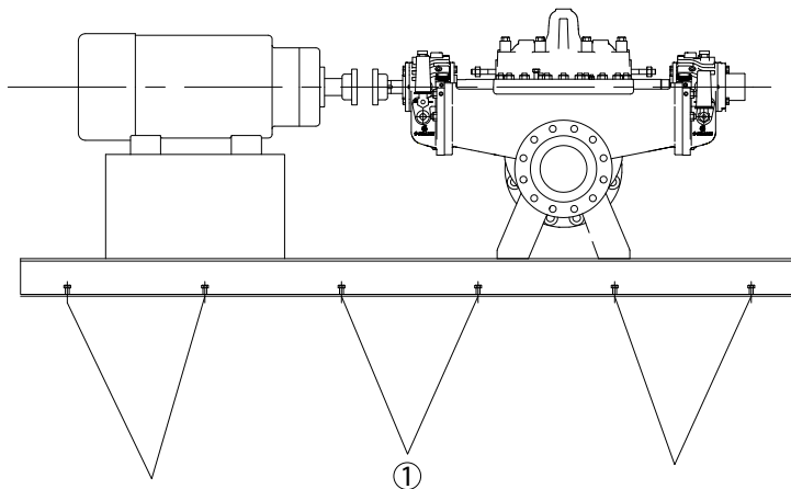
Figura 9: Ubicaciones de los tornillos elevadores, vista lateral
