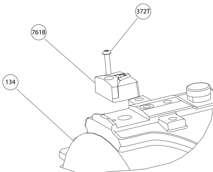
Figura 85: Sujeción del monitor de estado a la caja de rodamientos
