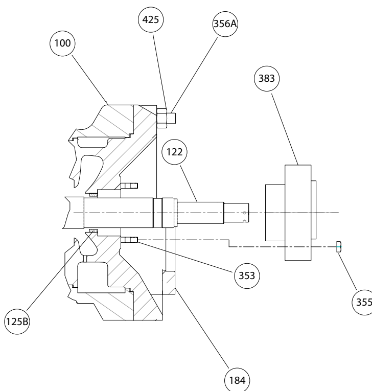
Figura 72: Monte el sello mecánico del cartucho en el extremo de empuje
