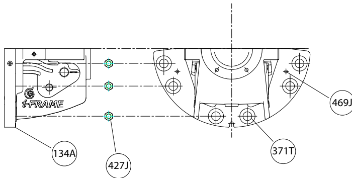
Figura 80: Ensamble la mitad inferior de bastidor de cojinetes
