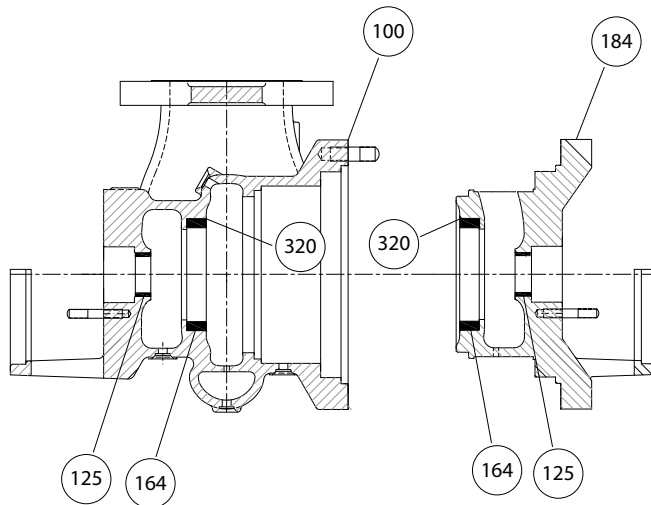
Figura 64: Reemplazamiento de los anillos y casquillo de desgaste
