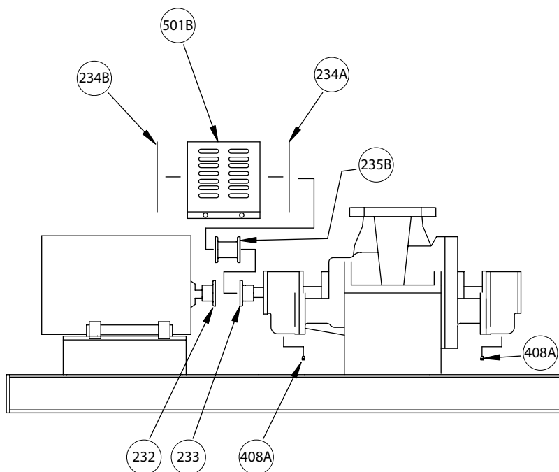
Figura 37: Conjunto del protector del acoplamiento
