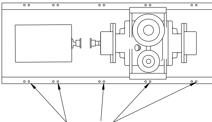
Figura 10: Ubicaciones de los tornillos elevadores, vista superior
