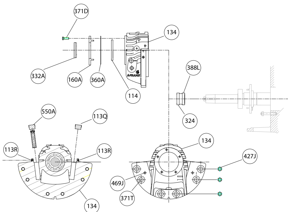
Figura 76: Ensamble del alojamiento de cojinetes radiales
