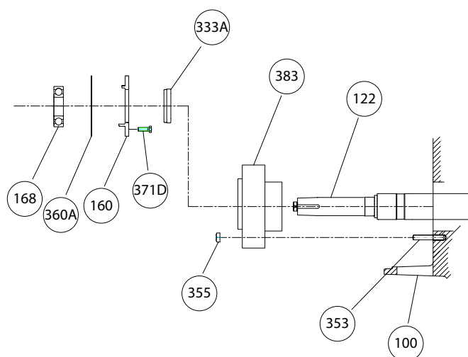
Figura 75: Ensamble del rodamiento radial
