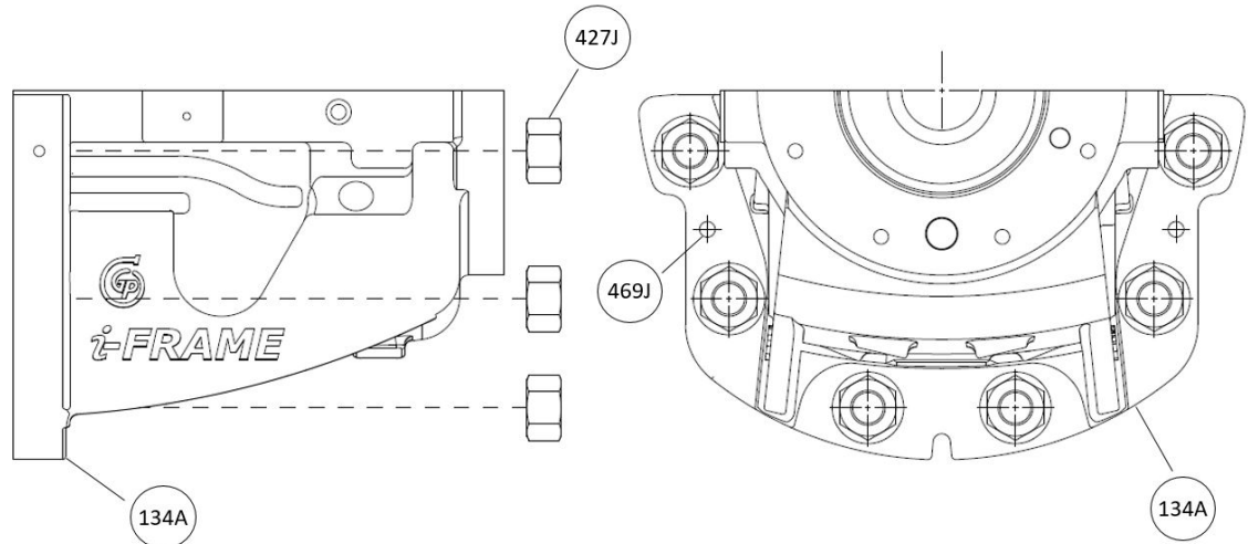
Figura 55: Extracción de la clavija de sujeción de empuje
