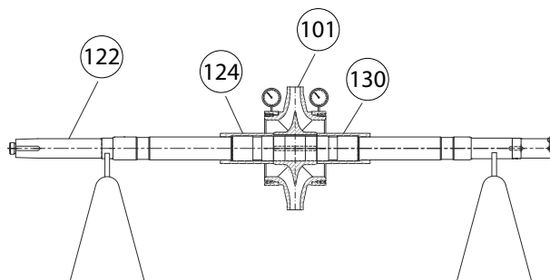
Figura 67: Inspecciones previas al montaje del rotor
