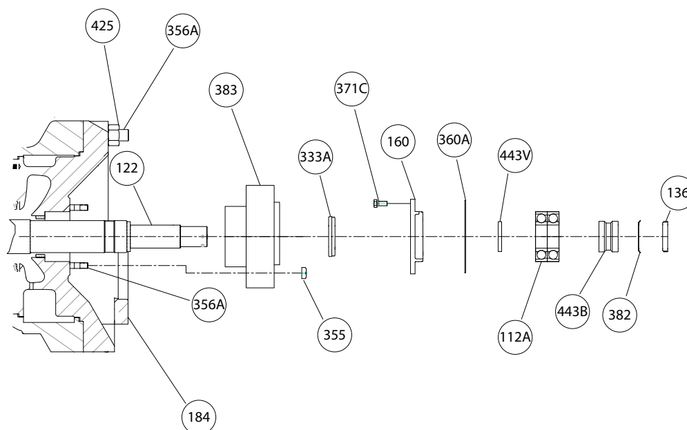
Figura 73: Montaje del cojinete de empuje
