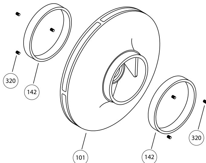
Figura 65: Reemplazamiento del anillo de desgaste
