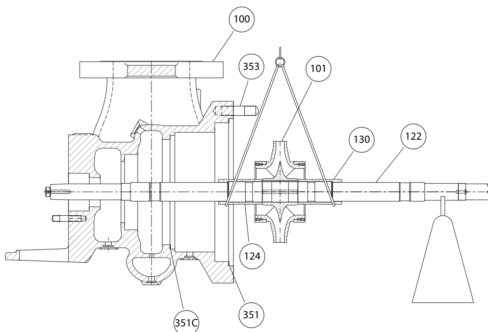
Figura 68: Levantamiento del elemento rotatorio con eslinga
