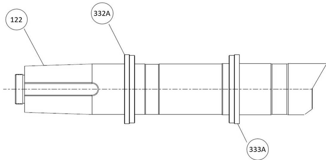
Figura 87: Instalación del sello laberinto radial interno
