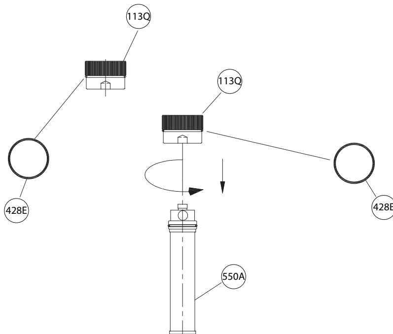
Figura 29: Instalación del filtro nuevo
