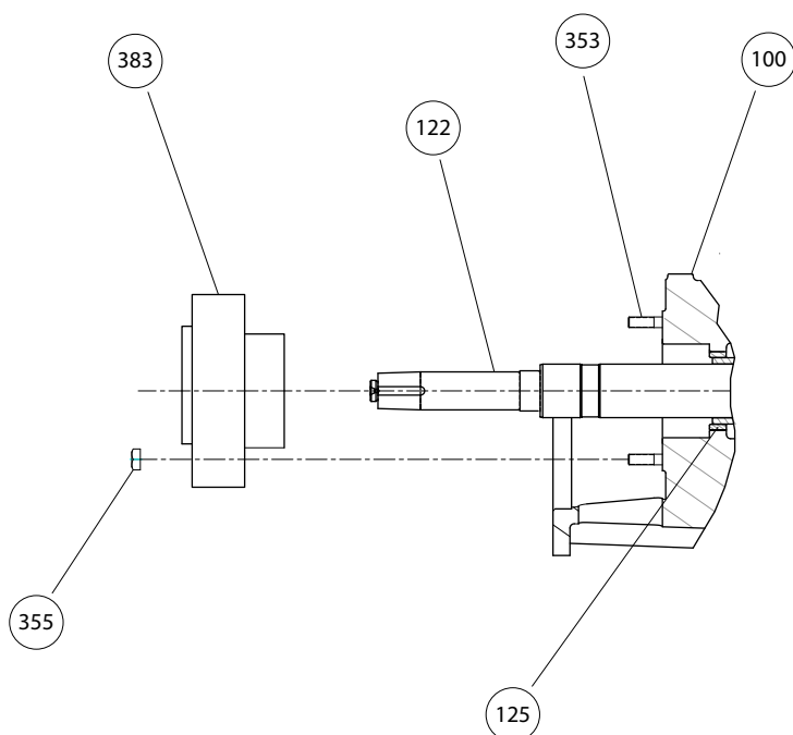
Figura 71: Monte el sello mecánico del cartucho en el extremo radial
