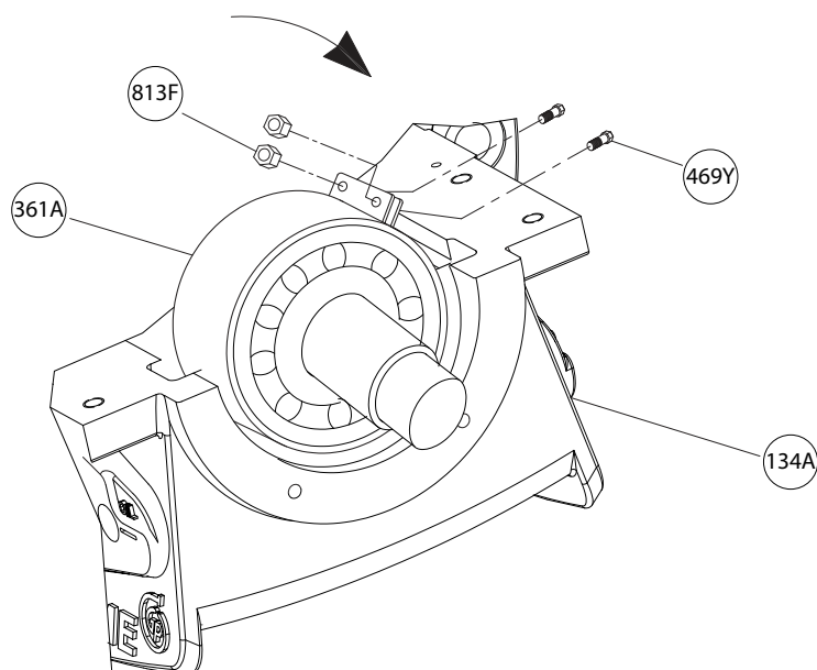
Figura 79: Instalación del retenedor del rodamiento
