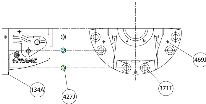
Figura 48: Extracción de la clavija de sujeción
