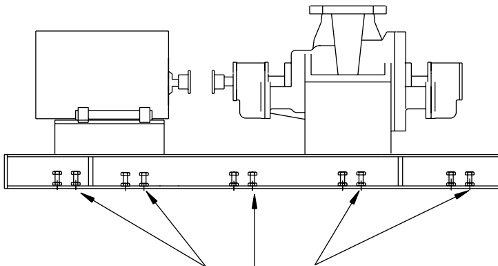
Figura 9: Ubicaciones de los tornillos elevadores, vista lateral
