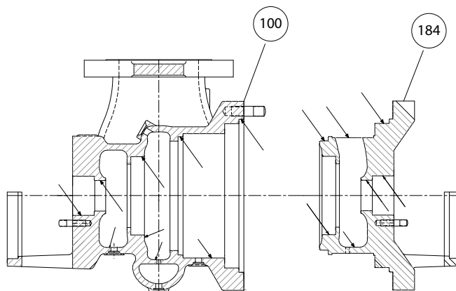
Figura 59: Inspección de la carcasa y el cabezal
