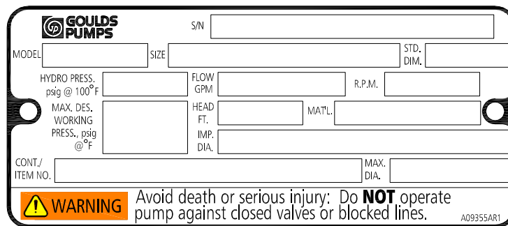
Figura 4: Placa de identificación en la carcasa de la bomba con unidades imperiales
