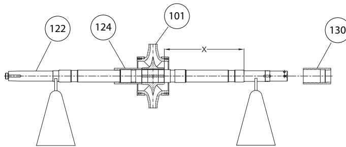
Figura 66: Conjunto del rotor
