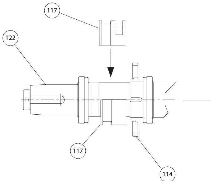
Figura 82: Conjunto de cojinete de manguito radial
