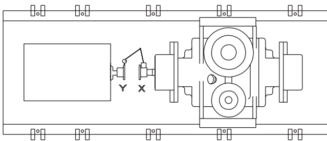
Figura 15: Ejemplo incorrecto de alineación horizontal (vista superior)
