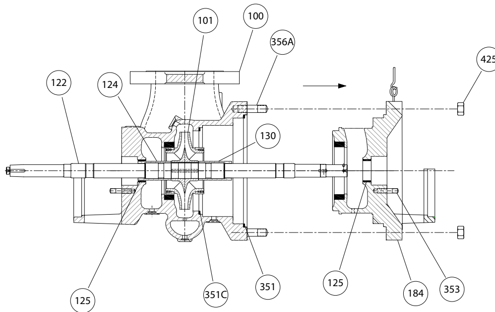
Figura 56: Eliminación del cabezal
