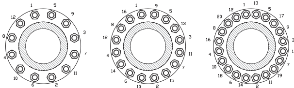
Figura 70: Marca de pasador
