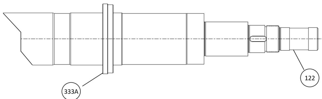
Figura 85: Instalación del sello laberinto de empuje interno
