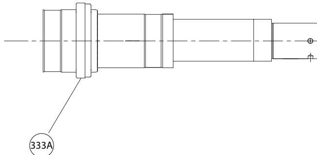
Figura 77: Instalación del sello de laberinto interior
