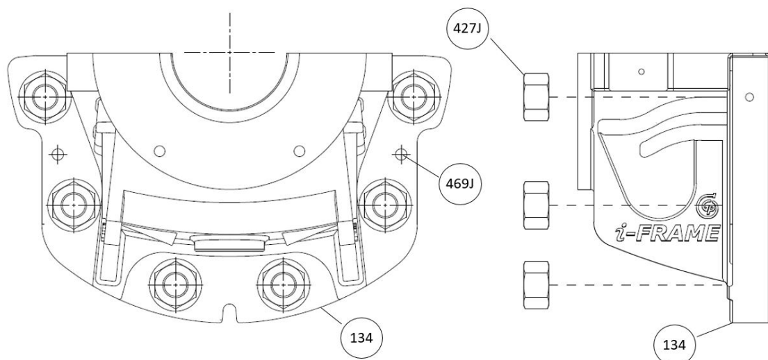
Figura 52: Extracción de la clavija de sujeción radial
