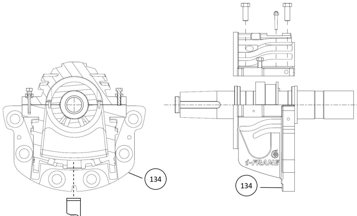
Figura 50: Desensamble el extremo radial (manga/esterilla para oscilación)
