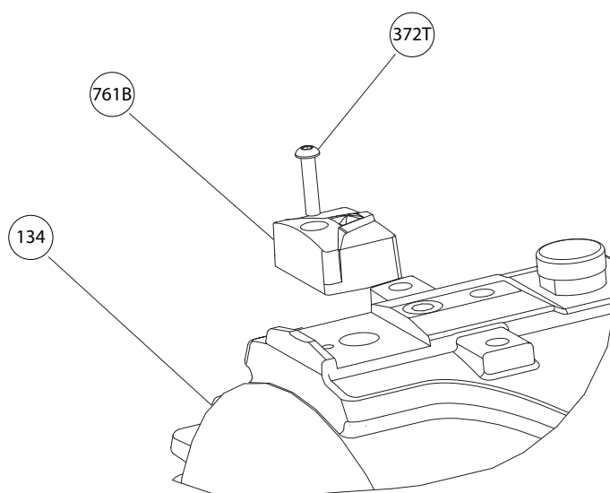
Figura 89: Sujeción del monitor de estado a la caja de rodamientos
