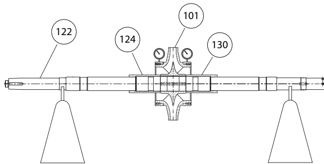
Figura 63: Rotor completamente ensamblado
