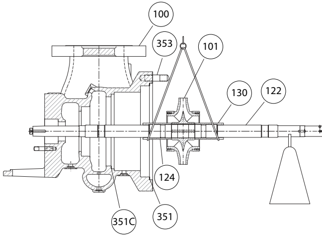
Figura 57: Levantamiento del elemento rotatorio con eslinga
