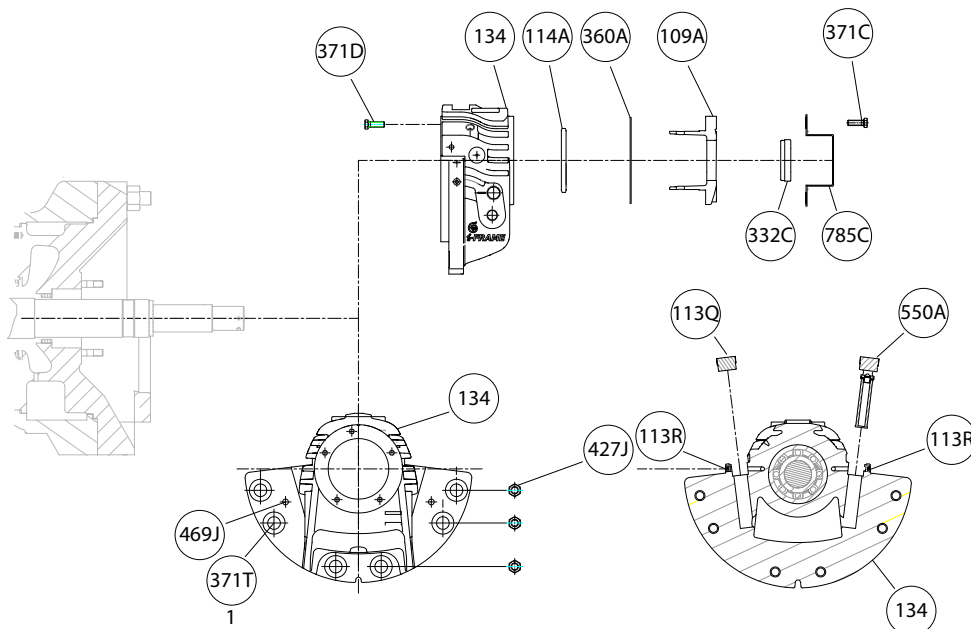
Figura 40: Desmontaje del bastidor de cojinete de empuje
