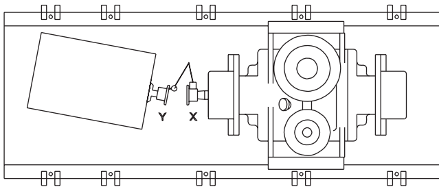
Figura 13: Ejemplo incorrecto de alineación horizontal (vista superior)
