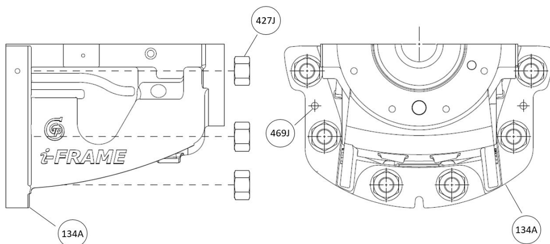
Figura 86: Ensamble el extremo de empuje
