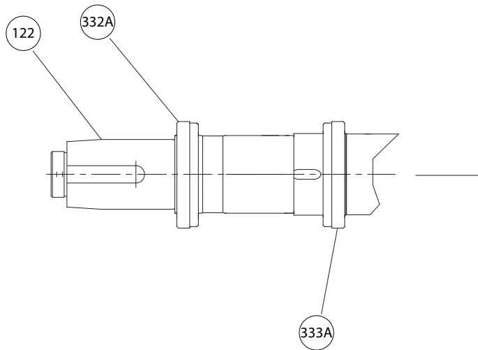
Figura 45: Extracción del sello laberíntico
