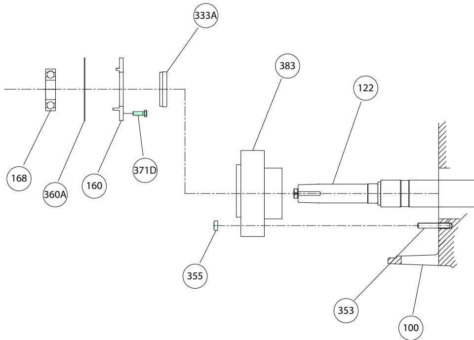
Figura 39: Extracción del cojinete radial
