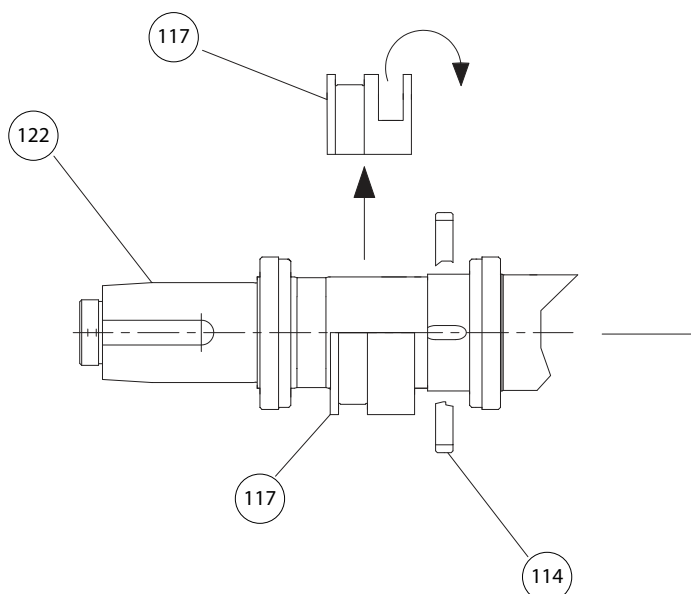
Figura 43: Retire el rodamiento del manguito radial
