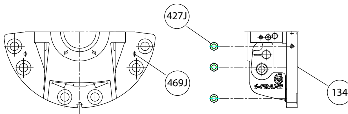
Figura 83: Instalación del alojamiento de rodamientos radiales
