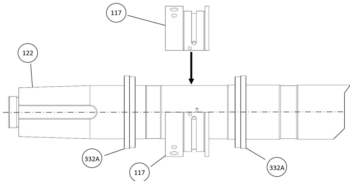
Figura 88: Conjunto de cojinete de manguito radial
