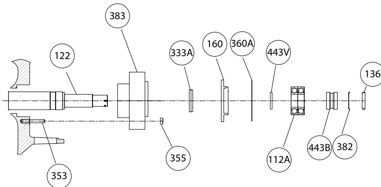
Figura 41: Desmontaje del cojinete de empuje
