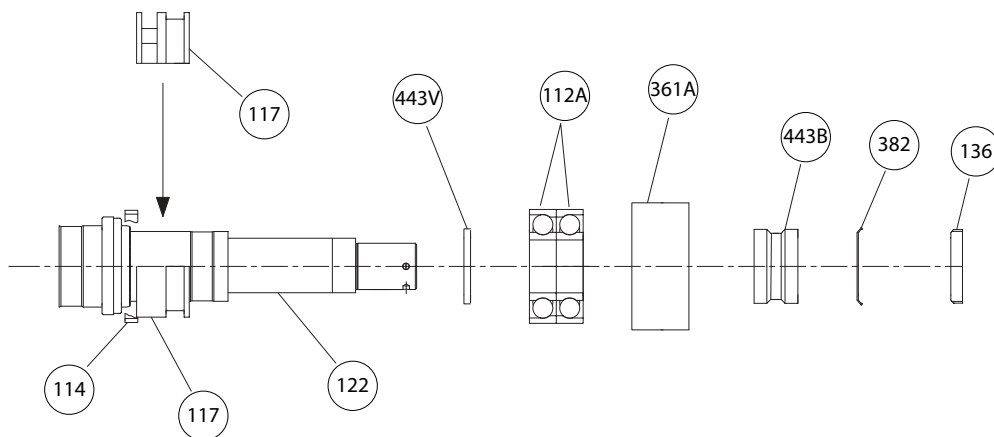
Figura 78: Montaje del manguito y cojinete de empuje
