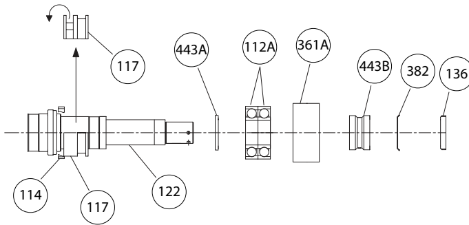
Figura 47: Extracción de cojinete del manguito y cojinete de empuje
