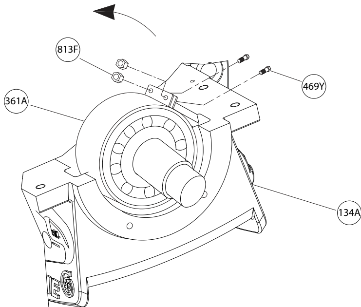
Figura 49: Extracción del retén del rodamiento
