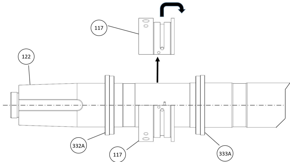
Figura 51: Extracción del cojinete de manguito radial
