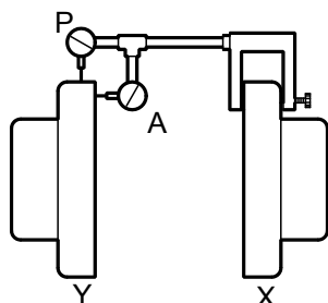
Figura 11: Acoplamiento del indicador de cuadrante
