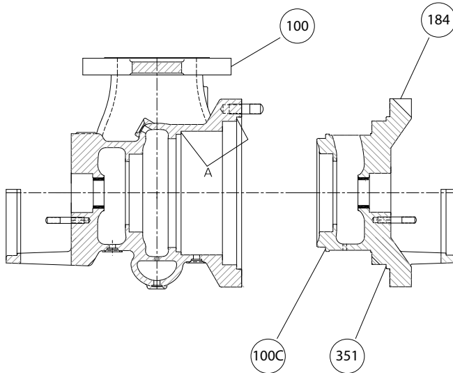
Figura 69: Montaje de juntas
