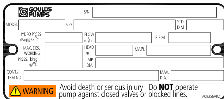
Figura 5: Placa de identificación en la carcasa de la bomba con unidades métricas
