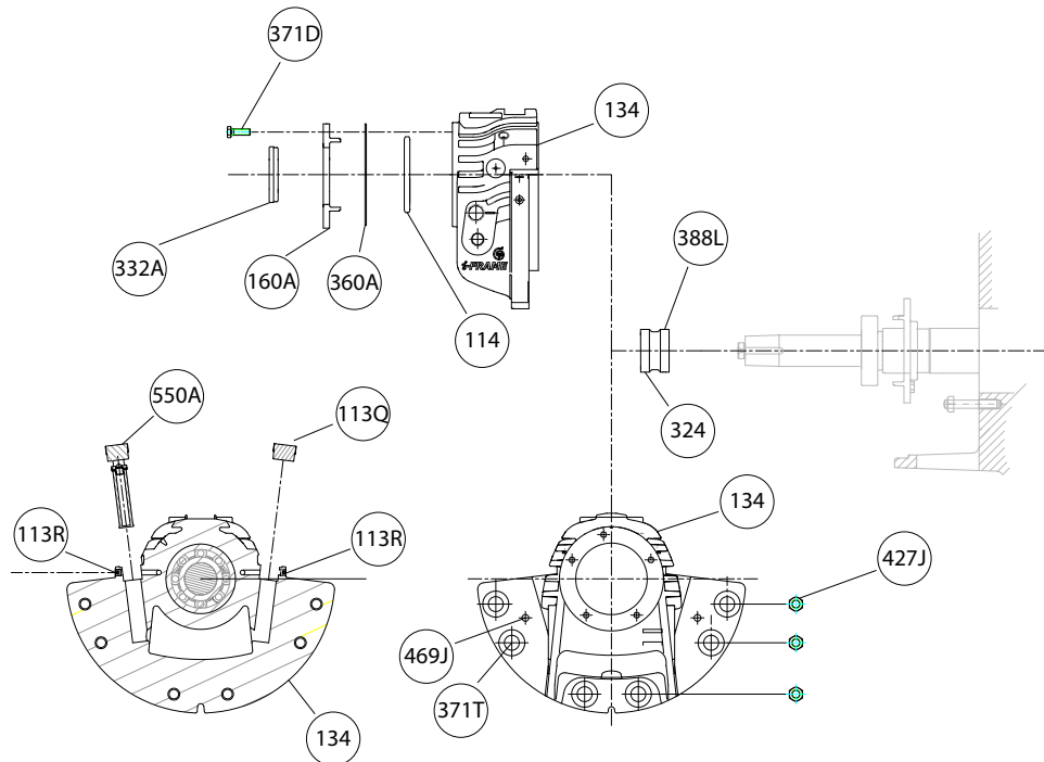
Figura 38: Ensamble del alojamiento de rodamientos radiales
