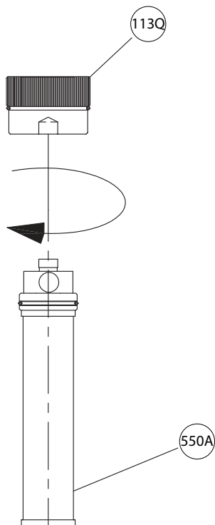
Figura 27: Desmontaje del filtro
