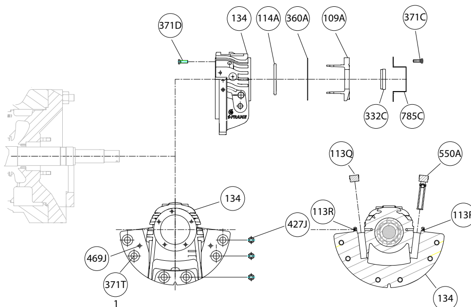
Figura 74: Montaje del bastidor de rodamientos de empuje
