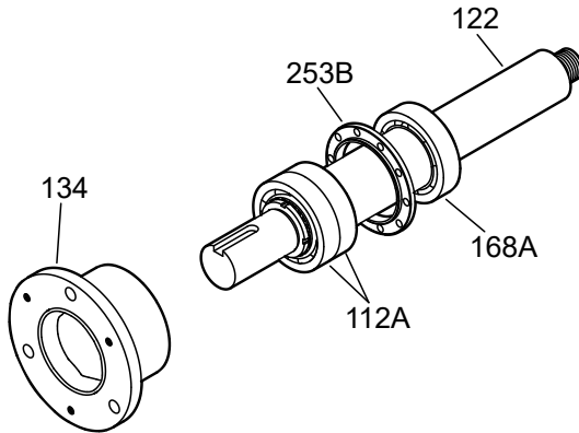
Şekil 98: Rulman yatağı yeniden montajı
