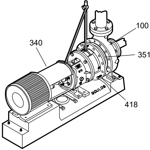
Şekil 31: C-yüzlü adaptör (340) örneği
