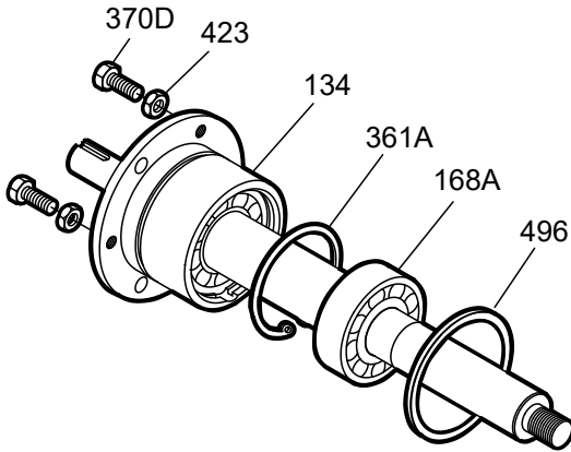
Şekil 65: Dış rulman tutucu bileziğinin çıkarılması
