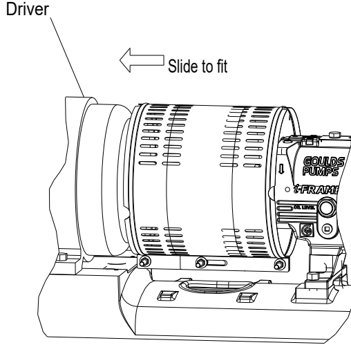
Şekil 44: Kaplin koruması tahrik birimi yarımını motora doğru kaydırın
