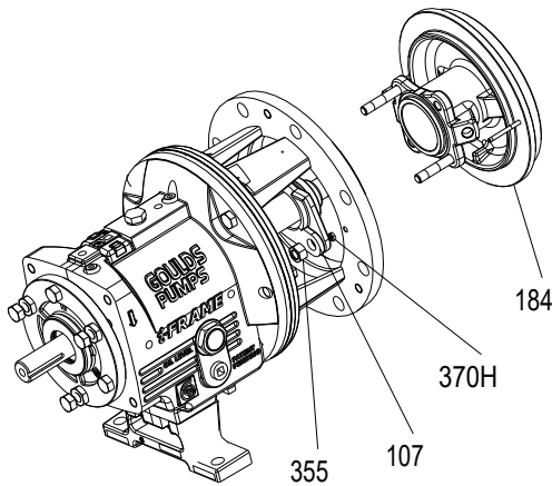
Şekil 60: Salmastra kutusu kapağının çıkarılması
