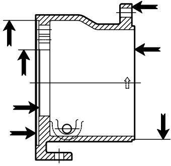
Şekil 85: C-yüzlü adaptör kontrol noktaları
