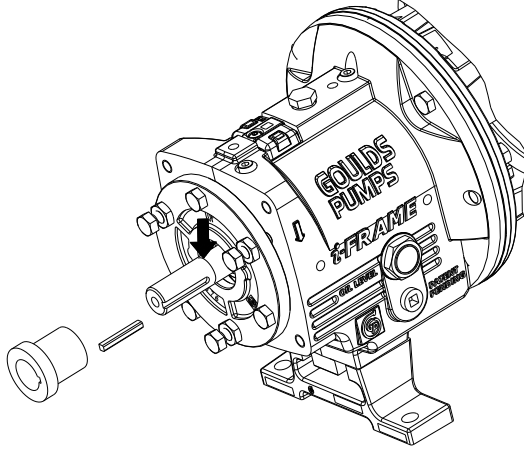
Şekil 53: Kaplin göbeğini çıkarma
