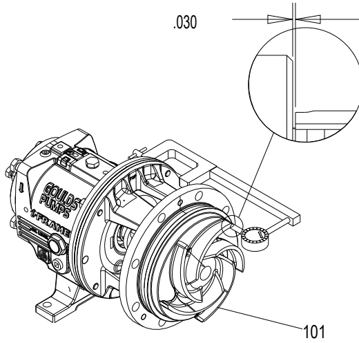
Şekil 126: Pervane salgısını kontrol edin
