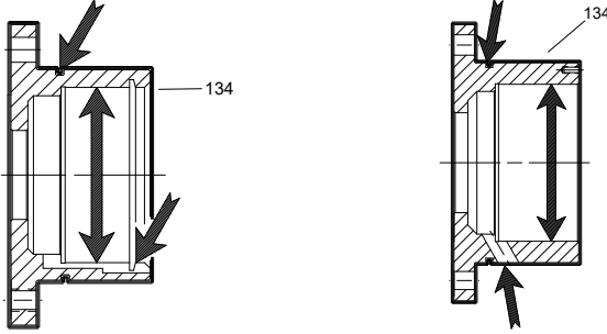
Şekil 89: STi ve MTi rulman ya- Şekil 90: LTi rulman yatağı tağı
