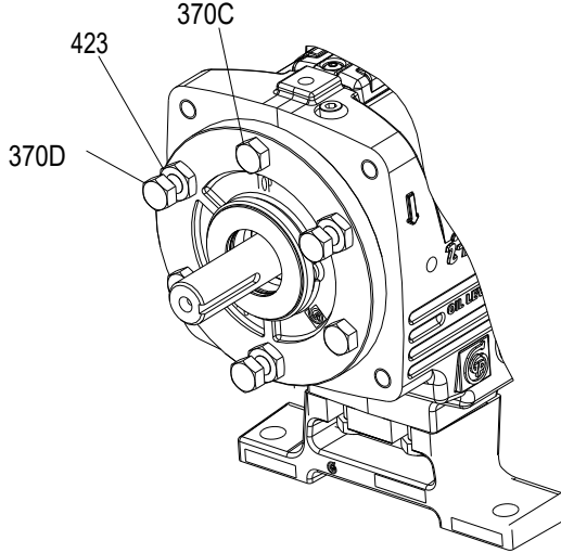
Şekil 127: Rulman yatağı üzerindeki kaskı cıvatalarını ve kriko cıvatalarını gevşetin.
