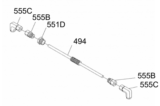
Şekil 136: Kanatçık borulu yağ soğutucu parça şeması
