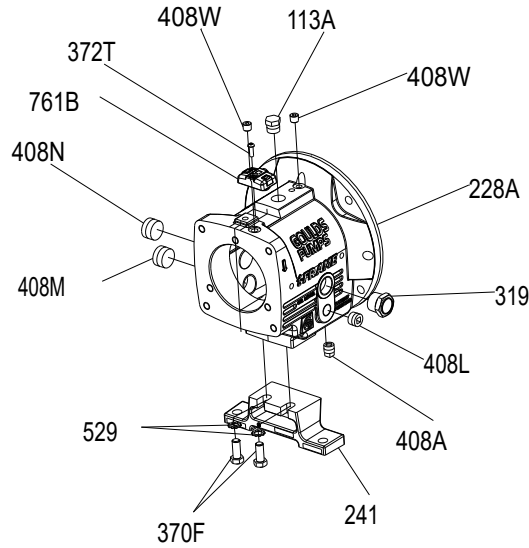
Şekil 131: İki yağ bağlantısını iki tapa ile birlikte yerine takın
