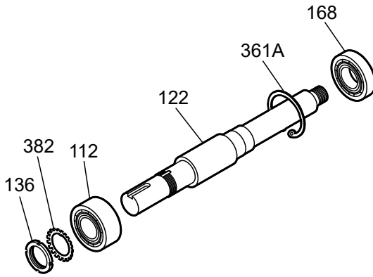
Şekil 67: Dış rulmanın çıkarılması
