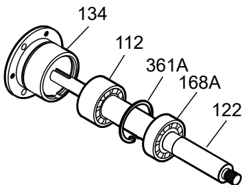
Şekil 66: Rulman yatağı ve rulmanların çıkarılması
