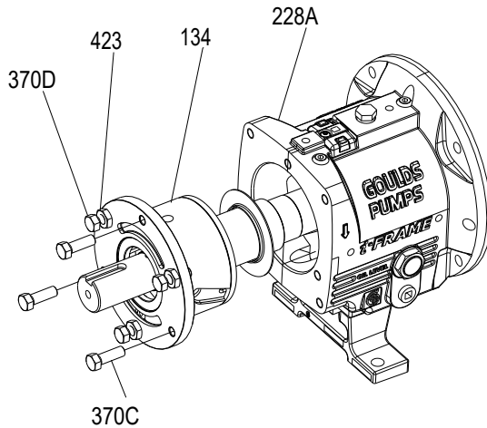
Şekil 73: Mil aksamının çıkarılması
