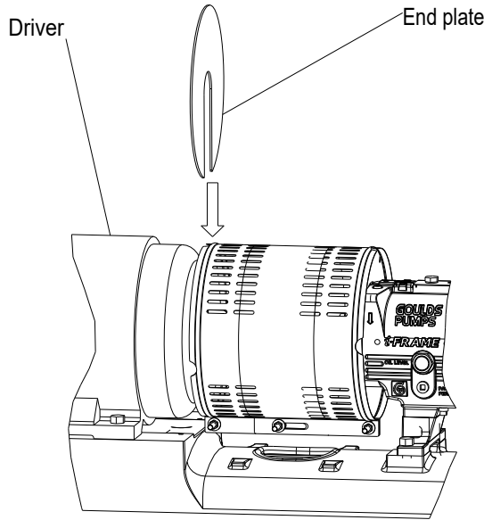
Şekil 43: Kaplin koruması yarımını yerleştirme
