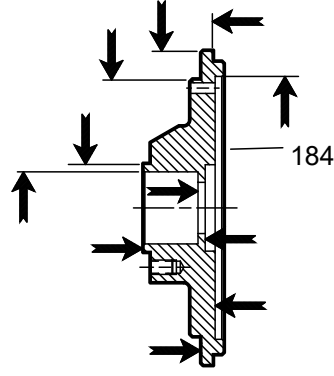
Şekil 87: Salmastra kutusu kapağı
