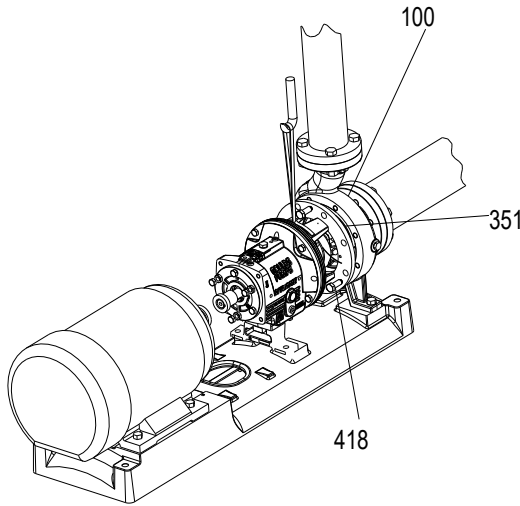
Şekil 128: Geri çekme düzeneğini kurun
