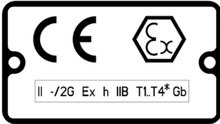
Şekil 15: Tipik Ex isim levhası
