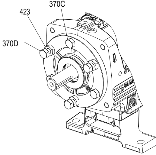
Şekil 125: Kaskı civatalarını gevşetin
