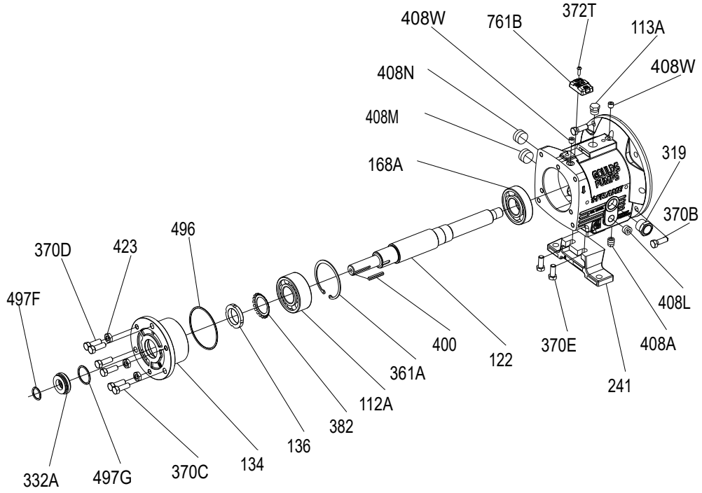
Şekil 134: MTi rulman gövdesi parça şeması
