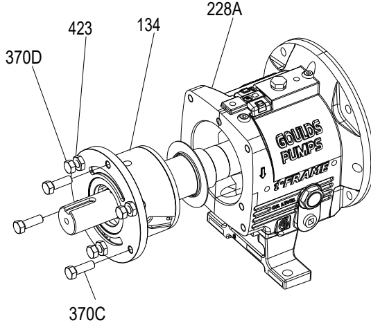
Şekil 64: Mil aksamının çıkarılması
