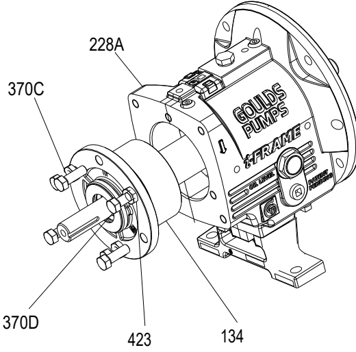
Şekil 94: Kriko civatası ve kilit somunun yeniden montajı
