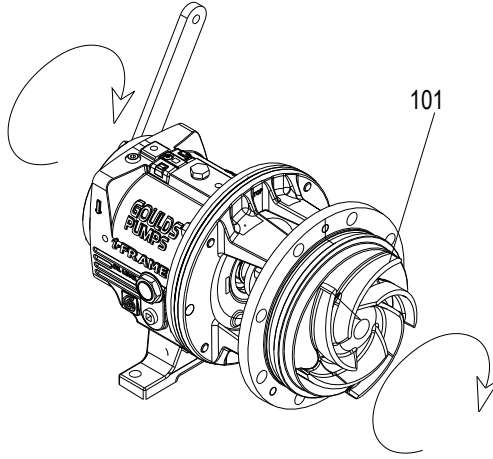
Şekil 124: Pervaneyi sıkın
