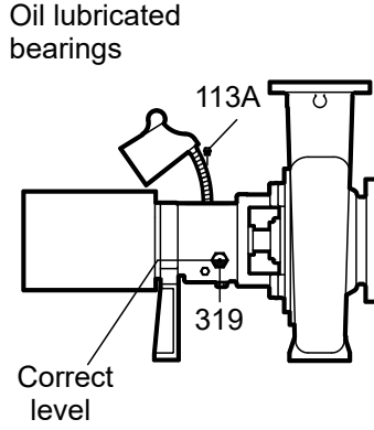
Şekil 45: Yağ doldurma bağlantısı
