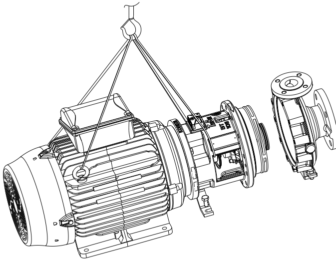
Şekil 52: Geri çekme tertibatı
