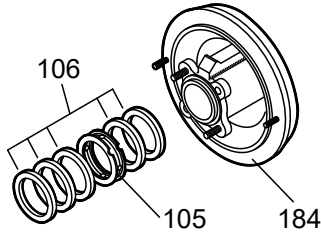
Şekil 62: Kutu ve sızdırmazlık bileziğinin çıkarılması
