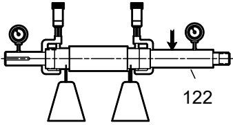
Şekil 81: Mil ölçüm kontrolü
