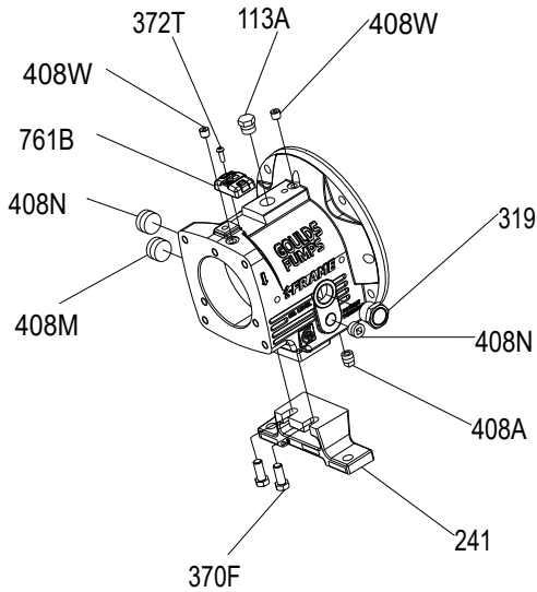
Şekil 78: Tapanın çıkarılması
