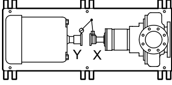
Şekil 30: Yanlış yatay hizalamanın üstten görünümü
