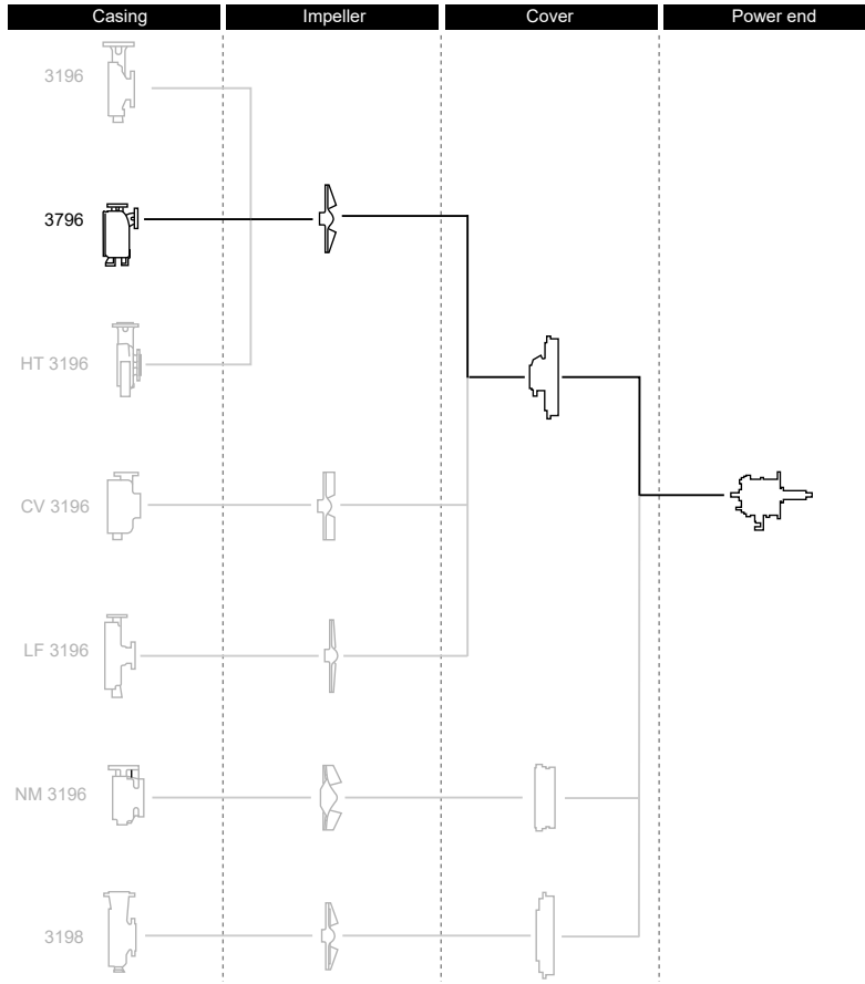
Şekil 11: 3796 parça tanımı
