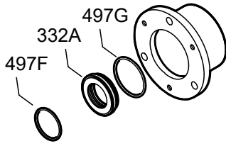
Şekil 72: Dış boğumlu yağ sızdırmazlık sökme
