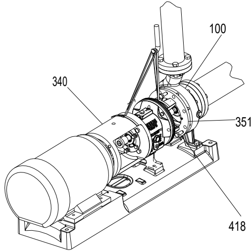
Şekil 51: Geri çekme tertibatını çıkarma (C-yüzlü adaptör olmadan)
