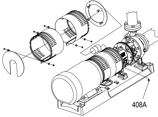
Şekil 49: Geri çekme tertibatını çıkarma (yağlamalı rulman yatağı)
