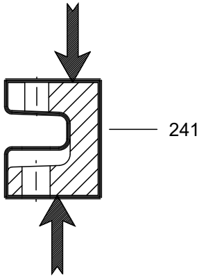
Şekil 84: Gövde ayak yüzeyi kontrol yerleri
