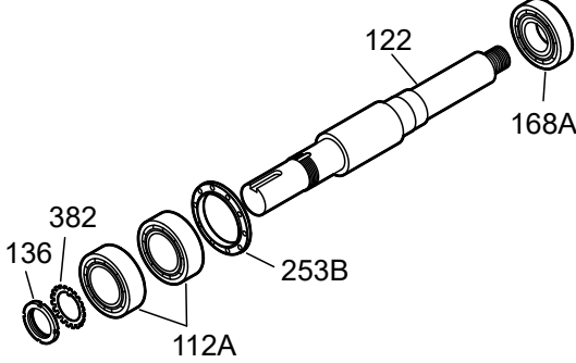
Şekil 97: İç rulman montajı
