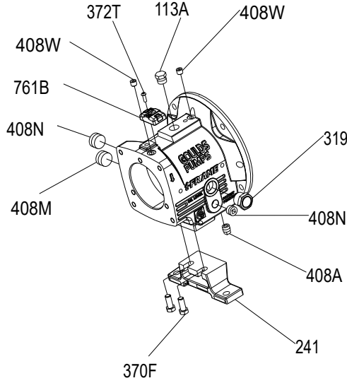
Şekil 95: Rulman gövde ayağının yeniden montajı
