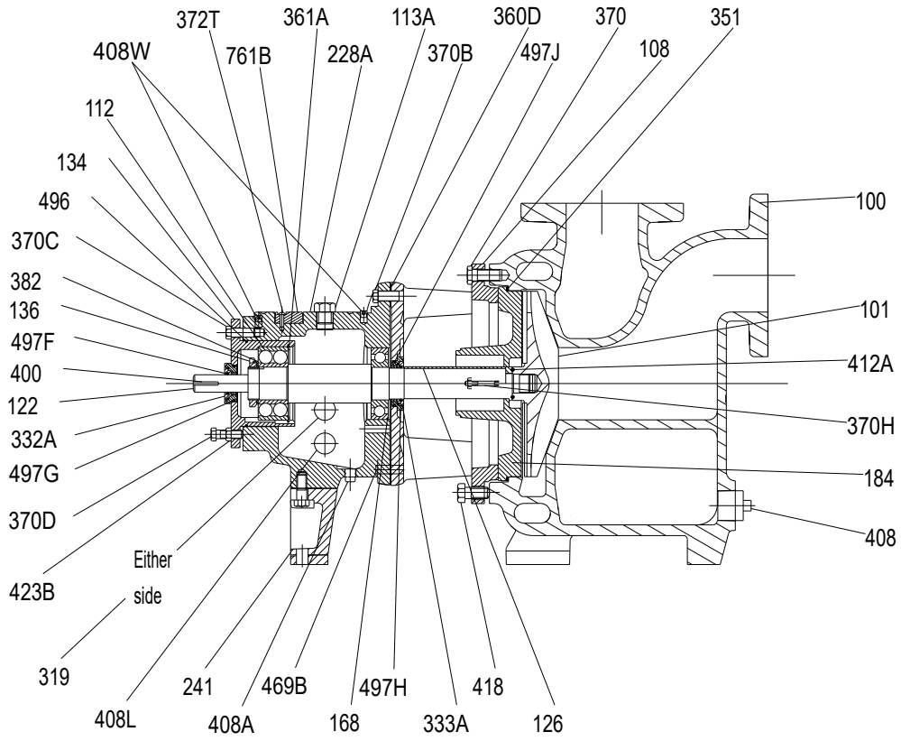
Şekil 132: 3796 çapraz kesit çizimi
