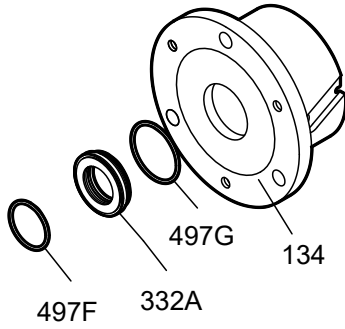
Şekil 77: O-ring sökme
