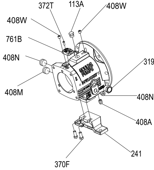
Şekil 91: Yağ buharı bağlantı tapası
