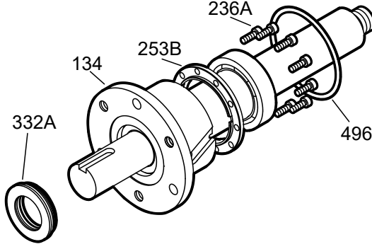
Şekil 104: Dış boğumlu yağ sızdırmazlık yeniden montajı
