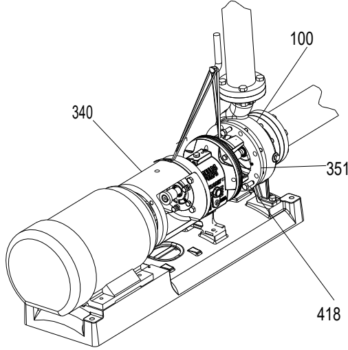
Şekil 129: Geri çekme düzeneğini kurun
