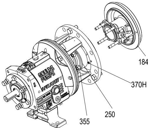
Şekil 58: Sızdırmazlık haznesi kapağının çıkarılması
