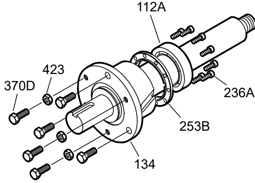
Şekil 74: Klempe halkasının çıkarılması
