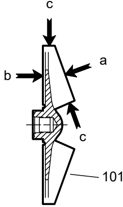
Şekil 80: Aşınma için kontrol edilecek alanlar 3196 çarkı.
