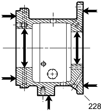
Şekil 83: Rulman gövdesi yüzey kontrol yerleri
