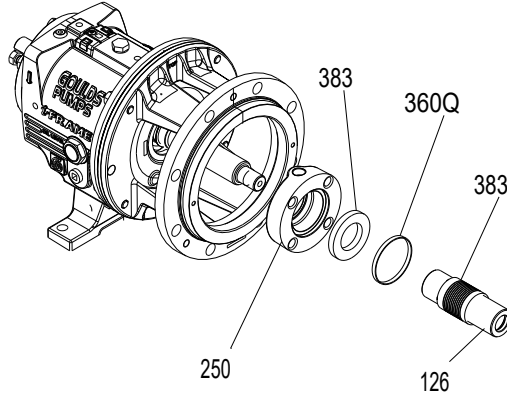
Şekil 59: Salmastra bileziğinin çıkarılması
