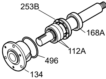
Şekil 75: Rulman yatağı ve rulmanın çıkarılması
