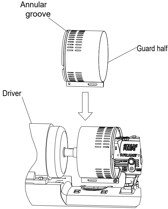
Şekil 42: Kaplin koruması yarımını yerleştirme
