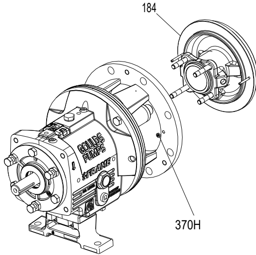
Şekil 117: Sızdırmazlık haznesi kapağı veya taban plakası montajı
