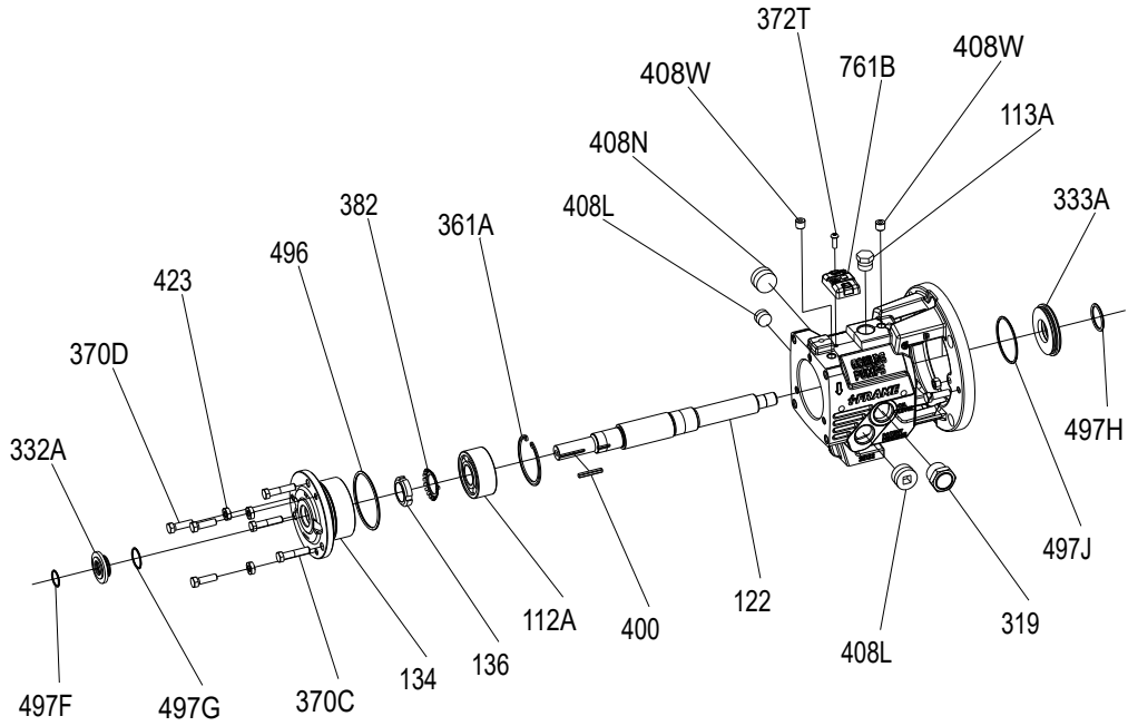
Şekil 133: STi rulman gövdesi parça şeması
