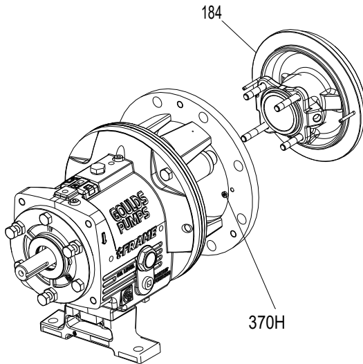
Şekil 114: Sızdırmazlık haznesini monte edin
