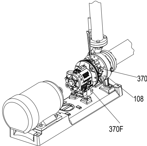
Şekil 50: Geri çekme tertibatını çıkarma (C-yüzlü adaptör ile)
