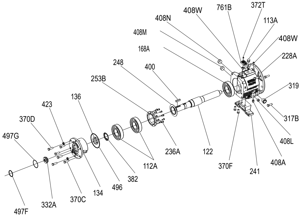
Şekil 135: LTi rulman gövdesi parça şeması
