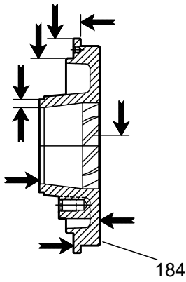
Şekil 88: TaperBore™ Plus
