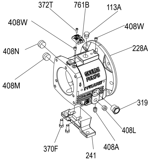
Şekil 100: Rulman gövde ayağını takın
