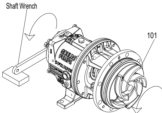
Şekil 54: Pervaneyi gevşetin
