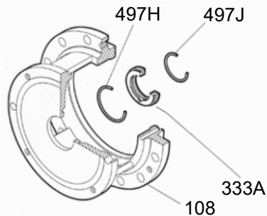
Şekil 63: O-ring sökme
