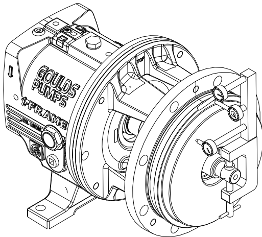
Şekil 118: Sızdırmazlık haznesi kapak kaçıklığını kontrol edin
