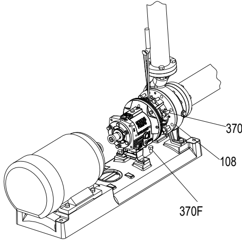
Şekil 130: Muhafaza vidalı krikolarını takın ve sıkın
