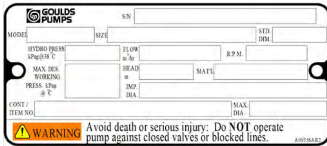
Şekil 13: Metrik birimler - pompa gövdesindeki isim plakası
