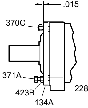
Şekil 36: Pervane boşluğu ayarı
