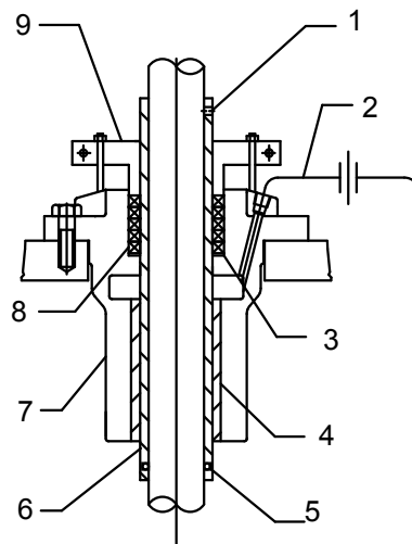
Abbildung 4: Stopfbuchse Typ A
