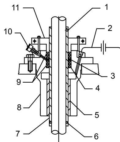
Figura 5: Caixa de espanque do tipo B
