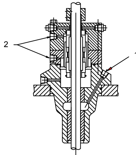
Figura 7: Selo montado em tandem (duplo não pressurizado)
