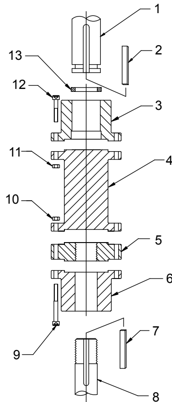
Figura 9: Acoplamento do tipo não espaçador
