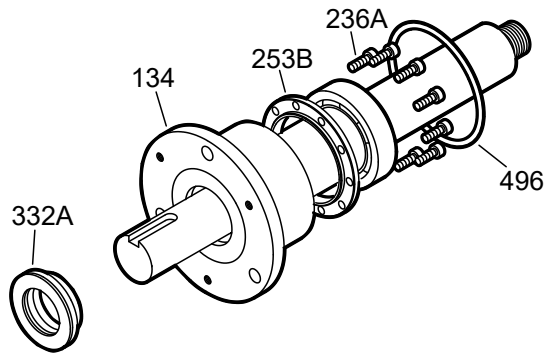
Figura 92: Reensamblaje de los sellos de aceite de laberintos externos
