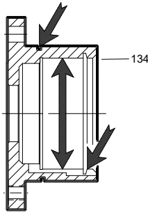
Figura 83: Porta-rodamientos STi y MTi
