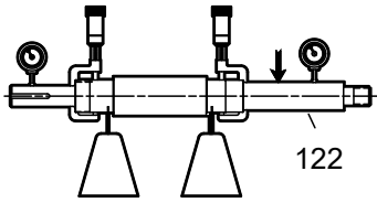
Figura 76: Control de las medidas del eje
