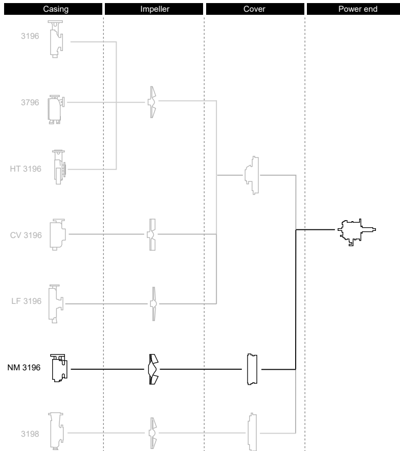
Figura 11: descripción de las piezas del modelo NM 3196
