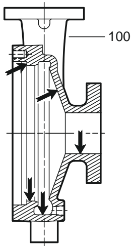
Figura 74: 3196, HT 3196, LF 3196, NM 3196 y carcasa 3198
