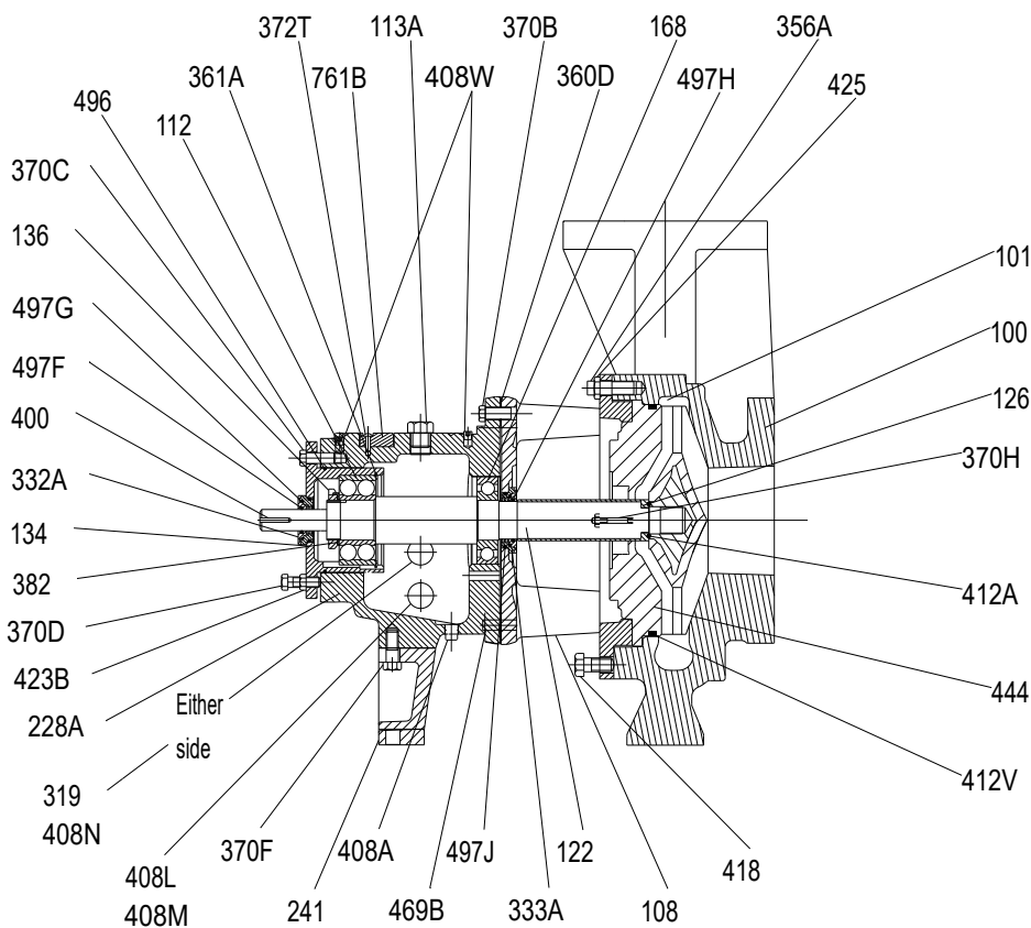
Figura 116: Plano de la sección transversal del modelo NM 3196
