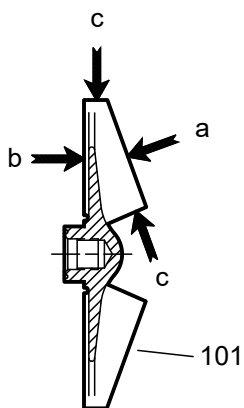
Figura 75: Áreas para inspeccionar el desgaste el impulsor 3196* ** .
