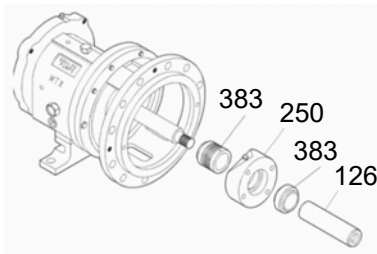
Figura 61: Quite el asiento estacionario y el prensaestopas
