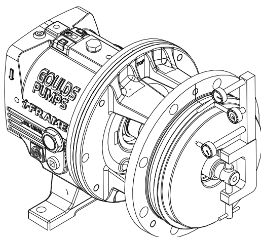
Figura 104: Controle el descentramiento de la cubierta de la cámara del sello
