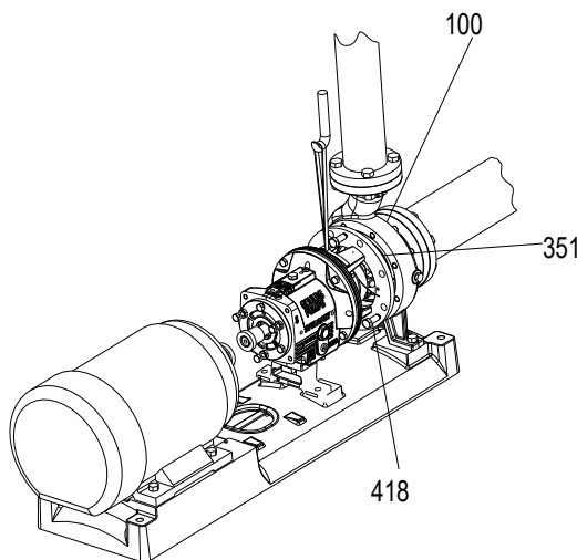
Figura 112: Instalación del conjunto de desmontaje posterior
