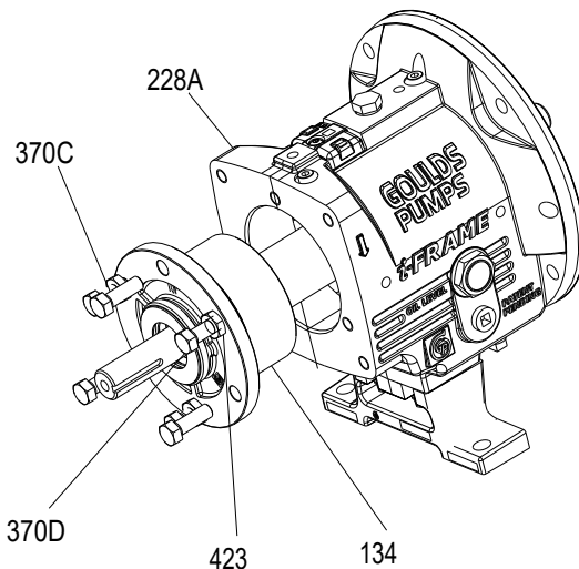
Figura 87: Reensamblaje de los pernos de extensión y de las tuercas de sujeción
