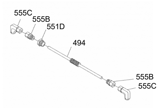
Figura 119: Vista detallada del enfriador de aceite del tubo con aletas
