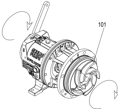
Figura 108: Ajuste el impulsor
