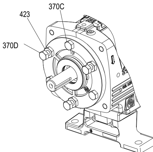
Figura 109: Afloje los pernos de sujeción
