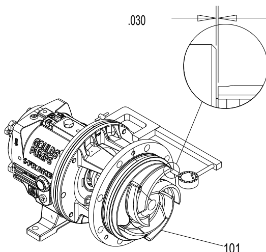
Figura 110: Verifique la desviación del impulsor
