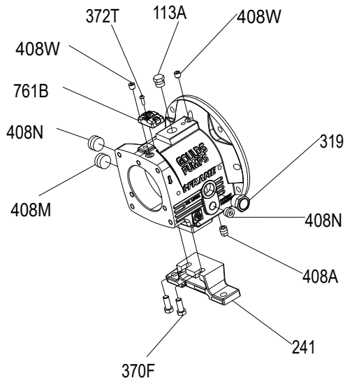
Figura 84: Tapones de la conexión de niebla de aceite
