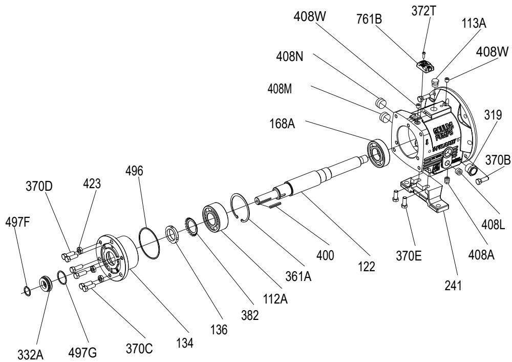
Figura 118: Vista detallada de la caja de rodamientos MTi
