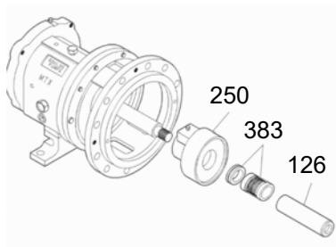
Figura 62: Extracción del asiento estacionario y de la cámara de sellado
