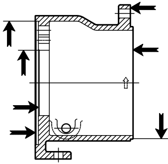
Figura 80: Ubicaciones de inspección del adaptador de cara C
