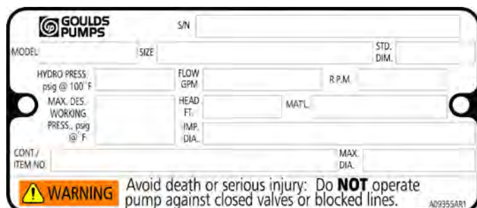
Figura 12: Placa de identificación en la carcasa de la bomba con unidades imperiales
