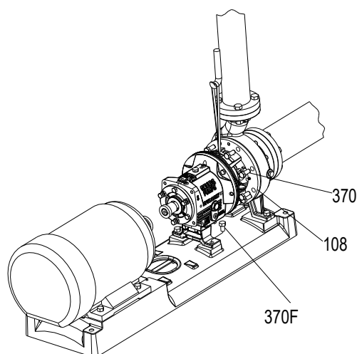
Figura 114: Instale y apriete los tornillos de sujeción de la carcasa.
