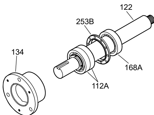
Figura 91: Reensamblaje de alojamientos de rodamientos
