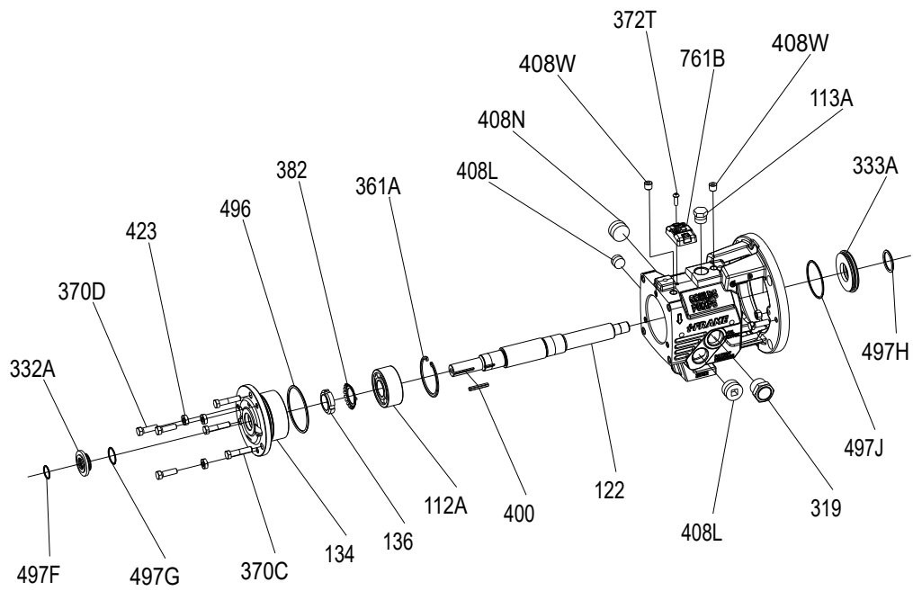
Figura 117: Vista detallada de la caja de rodamientos STi
