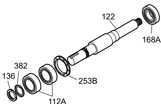
Figura 90: Reensamblaje de rodamientos internos
