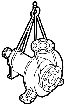
Figura 3: Ejemplo de un método de elevación adecuado
