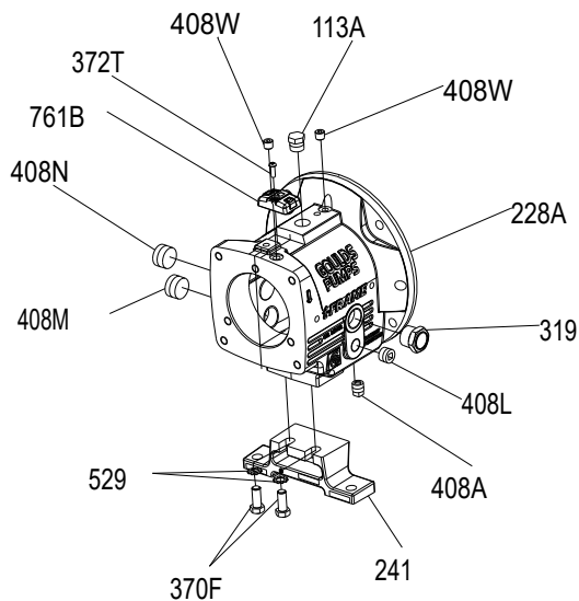
Figura 115: Reemplace dos accesorios de engrase con dos tapones
